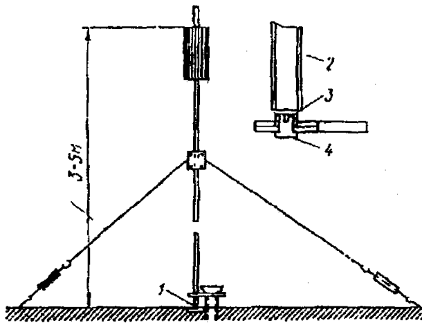
Рис. 31. Съёмная металлическая веха с визирным цилиндром 1 — центр пункта; 2 — веха; 3 — отверстие (центр пункта); 4 — болт
