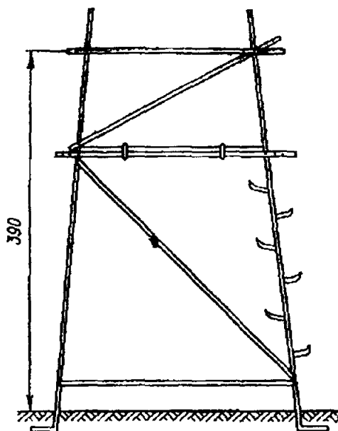
Рис. 27. Металлическая переносная площадка для наблюдения с пирамид-штативов. Изготавливается из уголкового стали ( 50 \times 50 \times 5 и 35 \times 35 \times 4 )
