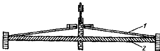
Рис. 29. Тур со съемной визирной целью 1 — кривизна; 2 — перекрытие (балка)
