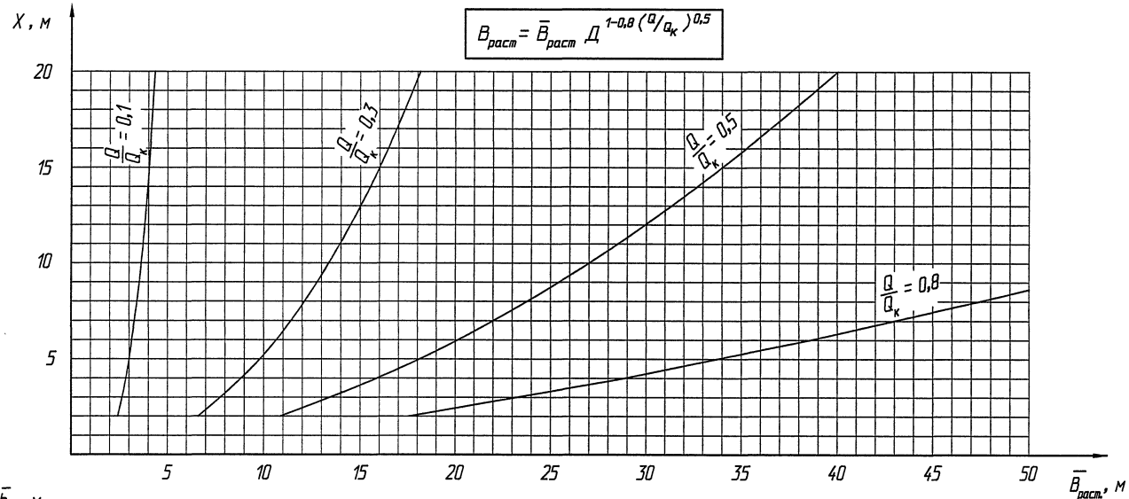
График 1 Определение ширины растекания потока
