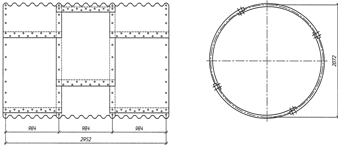
Секция трубы отв. 2,0 м
