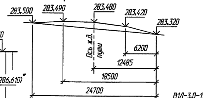
Схема строительного подъема
