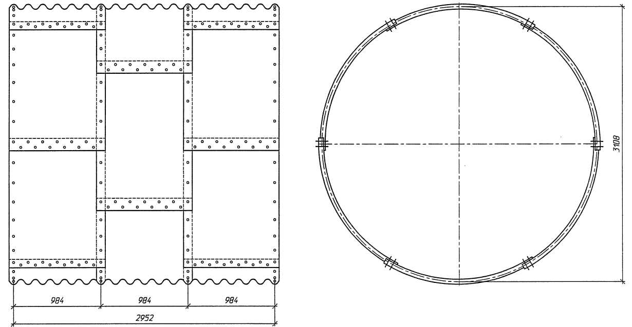
Секция трубы отв. 3,0 м
