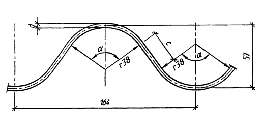
Гофр 164x57 мм
