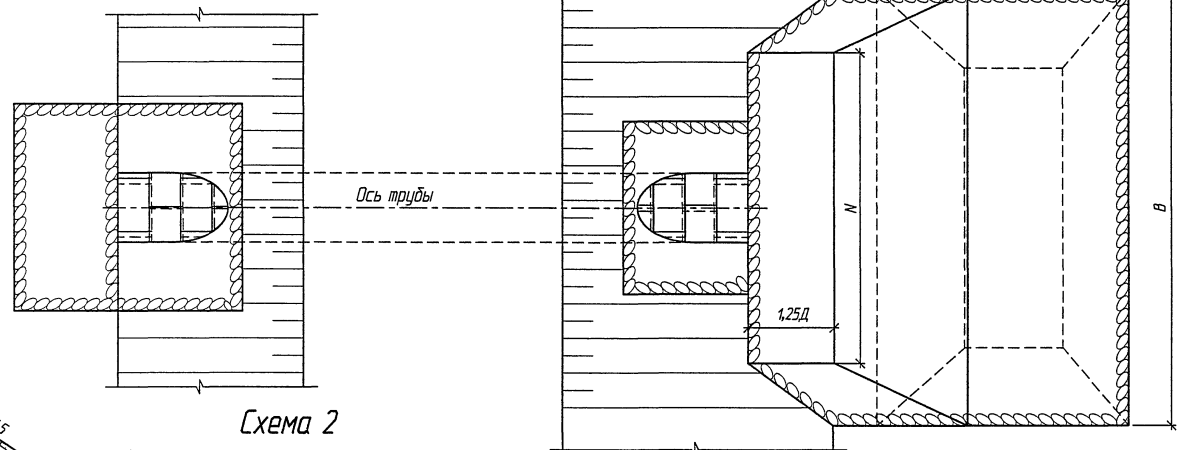
План
