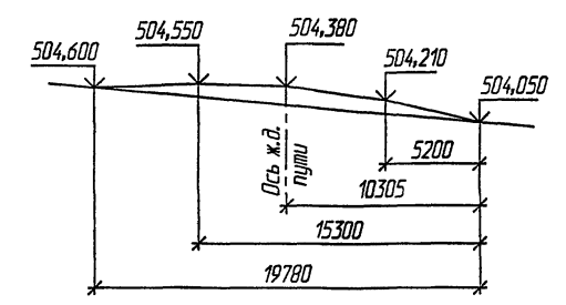
Схема строительного подъема
