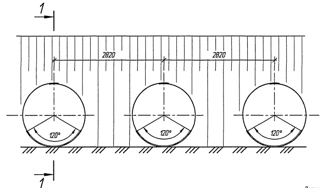
Фасад
