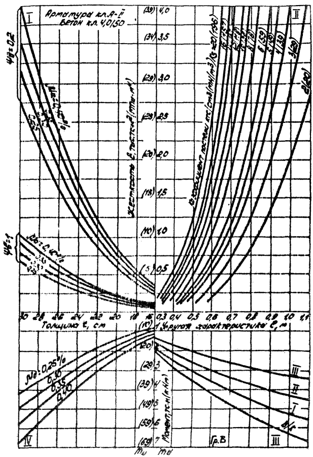
Рис. 15. Номограмма для расчета железобетонного покрытия группы участков В (для центральной части плиты)
