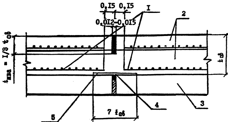
Рис. 4. Однослойное асфальтобетонное покрытие: I - стеклопластиковые сетки; 2 - слой усиления из асфальтобетона; 3 - существующее жесткое покрытие; 4 - побелка известковым молоком; 5 - пергамин
