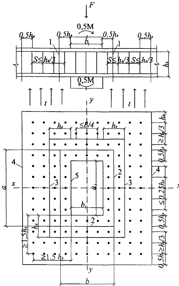
Рисунок 8.17 — Схема для расчета на продавливание железобетонной плиты с вертикальной равномерно распределенной поперечной арматурой при одностороннем огневом воздействии снизу плиты
