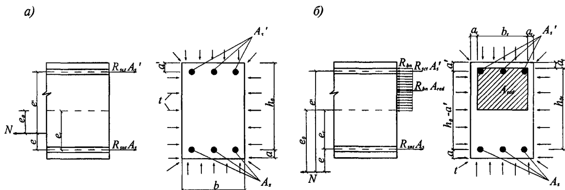
Рисунок 8.7 — Схема усилий и эпюра напряжений в сечении, нормальном к продольной оси внецентренно растянутого железобетонного элемента, при четырехстороннем обогриве во время пожара при расчете огнестойкости
