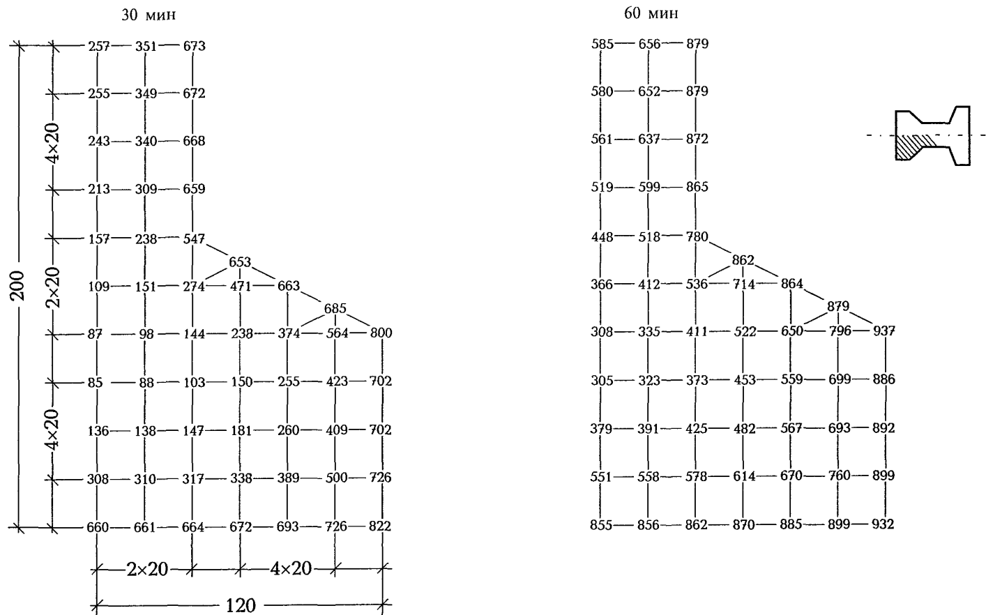
Рисунок Б.18 — Температура прогрева бетона в двутавровой балке со стенкой толщиной 80 мм и полкой шириной 240 мм при пожаре длительностью 30 и 60 мин
