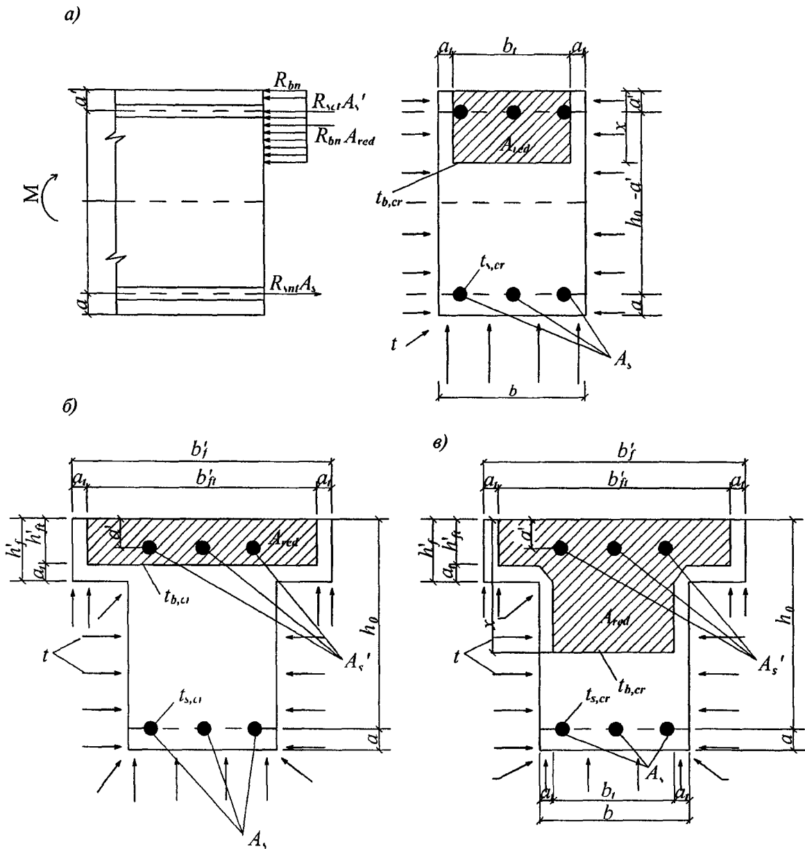
а — прямоугольного сечения, б — таврового сечения с сжатой зоной в полке; в — таврового сечения с сжатой зоной в ребре
