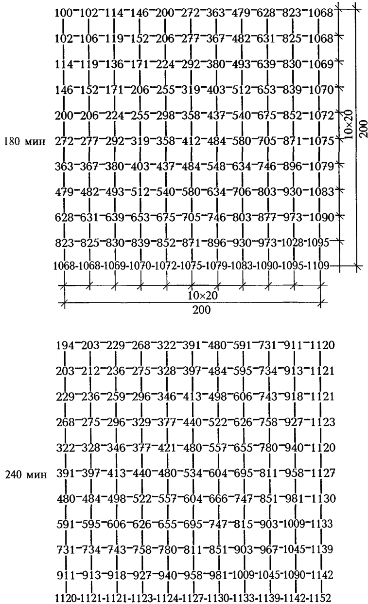
Рисунок Б.6 — Температура прогрева бетона в колонне сечением 400x400 мм при четырехстороннем воздействии пожара длительностью 180 и 240 мин
