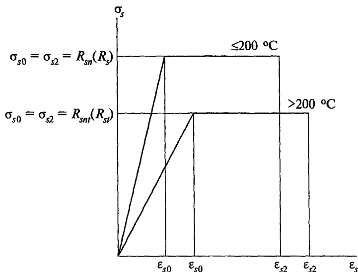
Рисунок 5.3 — Диаграмма деформирования арматуры при расчете огнестойкости и огнесохранности
