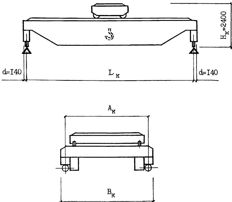
Рис.3. Основные габаритные параметры кранов
