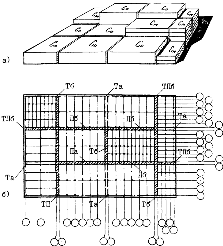
Рис. I. Здание, скомпонованное из разнотипных секций а) схематический общий вид; б) схематический план
