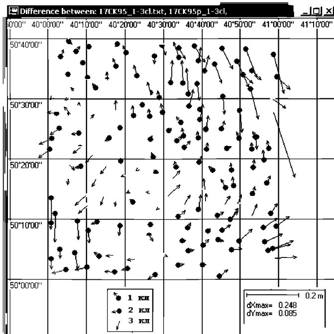
Рис. Пб.6. Остаточные расхождения координат пунктов ГТС 1-3 классов при ортогональном преобразовании для трапеции М3717
