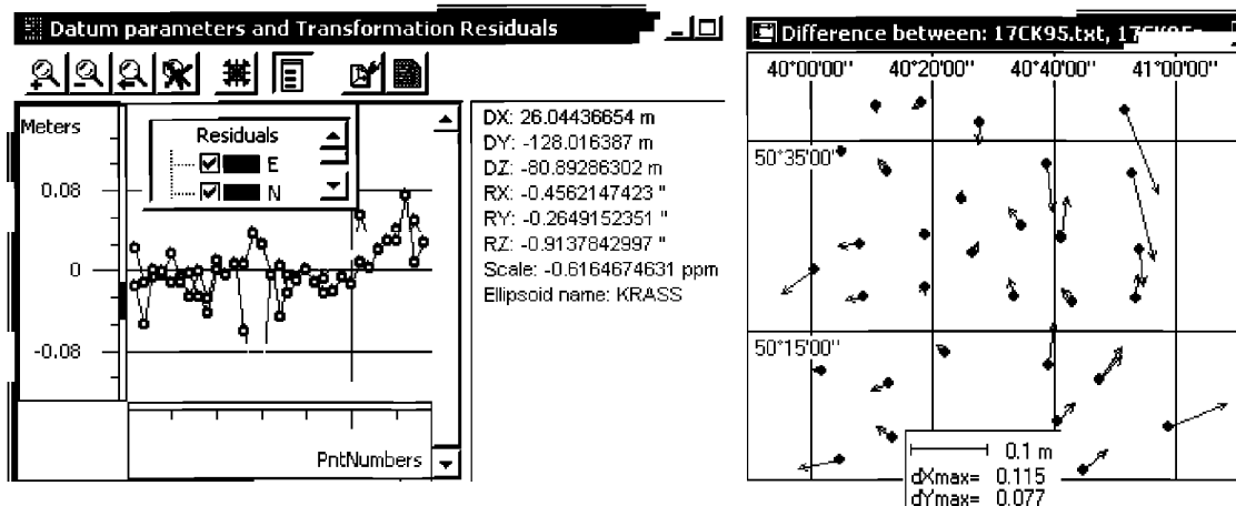
Рис. Пб.5. Определение параметров преобразования для трации М3717 и остаточные уклонения.
