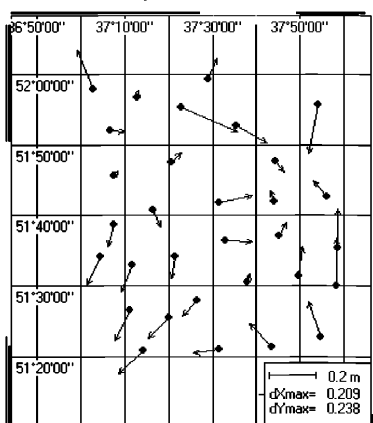
Рис. П6.4. Остаточные уклонения координат.
