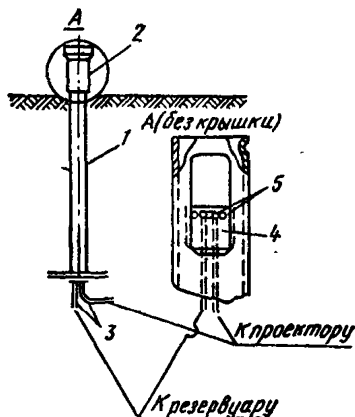
Рис. 38. Контрольно-измерительная колонка
