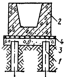
Рис. 5. Пример выполнения электроизоляционного разрыва в свайном фундаменте 1 — железобетонная свая; 2 — железобетонный ростверк; 3 — бетонная подготовка; 4 — слой асфальта
