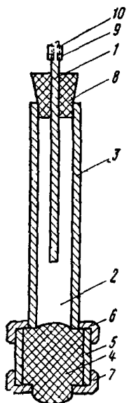
Рис. 20. Неполяризующийся медно-сульфатный электрод для контакта с бетоном
