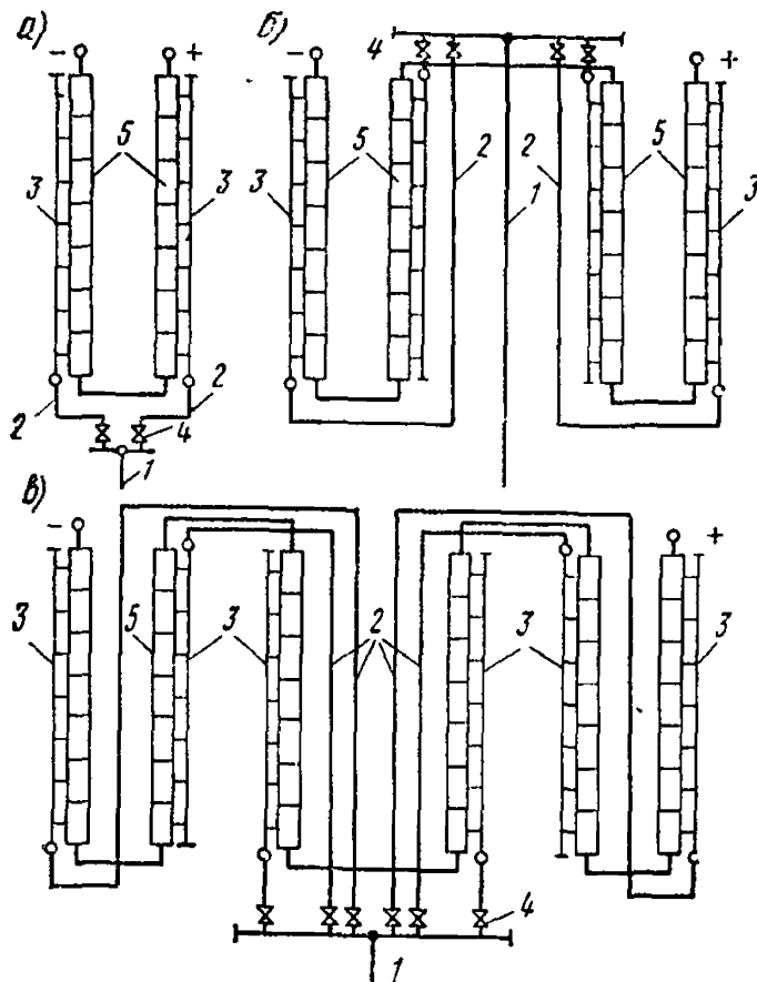
Рис. 17. Схема ввода электролитов в коллекторы электролизной установки, обладающая минимальными токами утечки
