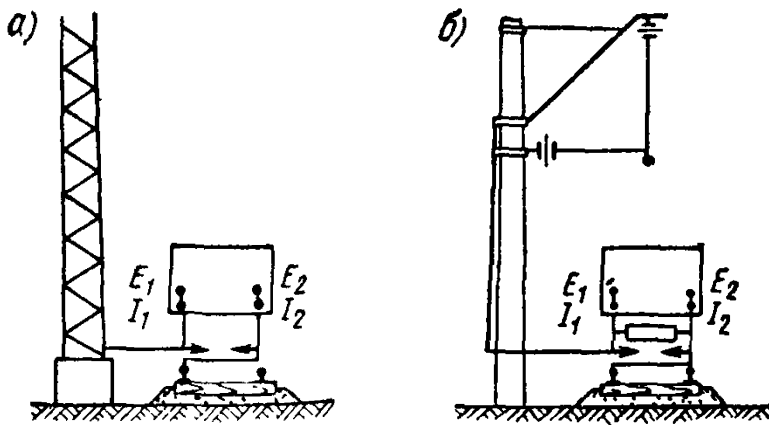
Рис. 22. Схемы измерения сопротивления цепи заземления опор в период эксплуатации R \leq 1000 \text{ Ом} (а) и R > 1000 \text{ Ом} (б) по двухэлектродной схеме
