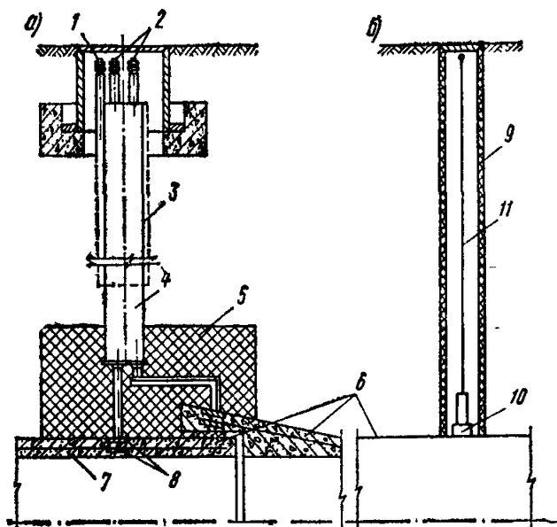
Рис. 11. Пример выполнения контрольно-измерительных пунктов для подземных железобетонных трубопроводов
