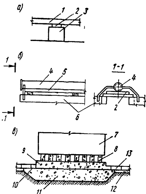
Рис. 2. Примеры конструкций из полимербетона для отделений электролиза водных растворов
