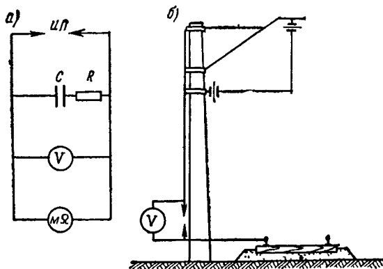
Рис. 27. Схемы проверки искрового промежутка перед установкой в цепь заземления (а) и в условиях эксплуатации (б)
