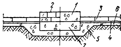
Рис. 3. Примеры фундаментов под оборудование (насосы, циркуляционные баки, опоры промывочных машин и т. д.) в отделениях электролиза водных растворов
