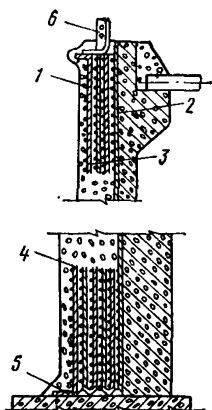
Рис. 10. Детали расположения основной, верхних и нижних контактных шин по отношению к кольцевой навивочной арматуре железобетонного резервуара
