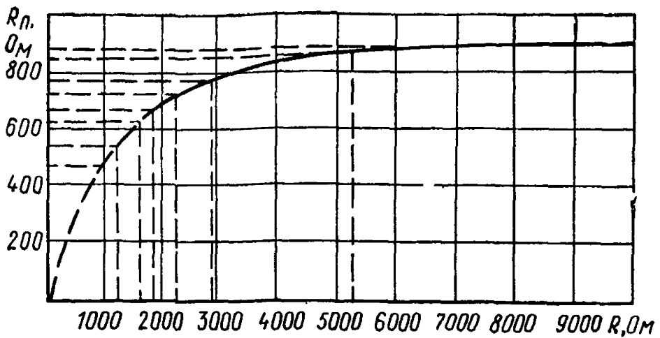
Рис. 23 Кривая для определения сопротивления цепи заземления опор по показаниям прибора при R_{доп} = 1000 \text{ Ом}
