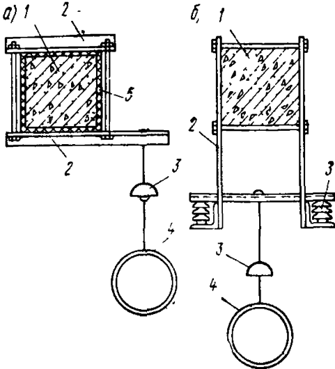
Рис. 14. Примеры выполнения металлических держателей для крепления трубопроводов
