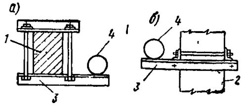
Рис. 13. Примеры выполнения держателей из электроизоляционных материалов для крепления трубопроводов
