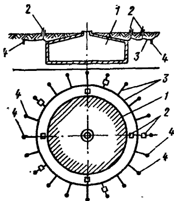
Рис. 37. Схема защиты железобетонного резервуара протекторными установками
