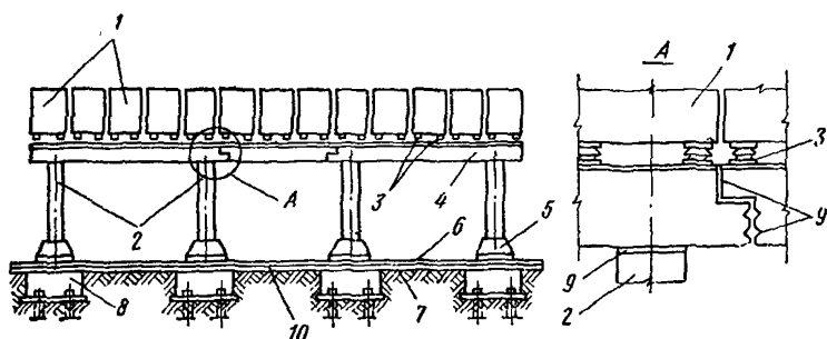
Рис. 1. Пример выполнения электроизоляционных швов в отделениях электролиза водных растворов
