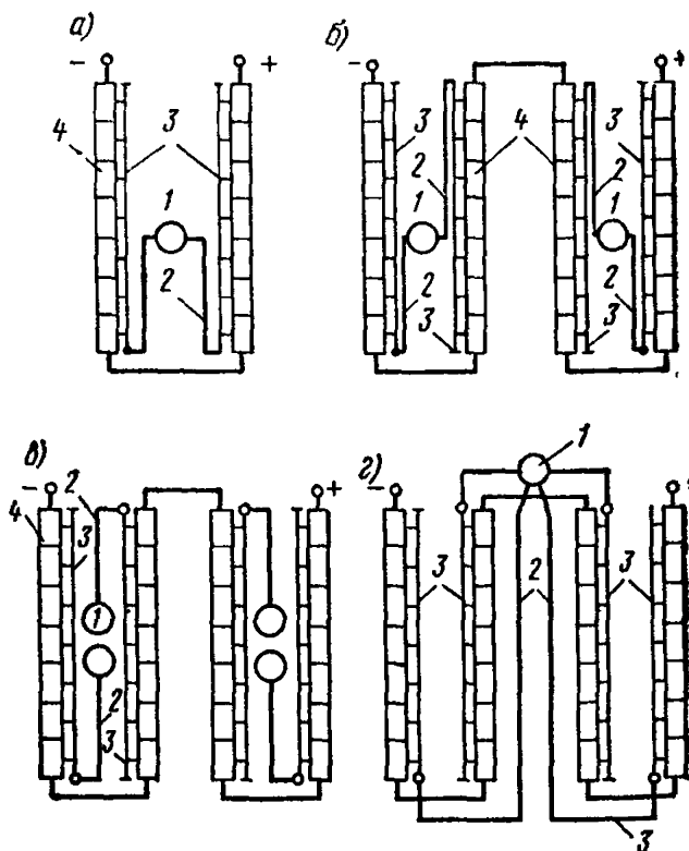
Рис. 18. Схемы присоединения технологического оборудования к электролизной установке с уменьшенными токами утечки
