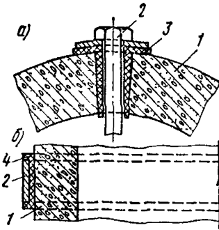
Рис. 6. Примеры изоляции деталей крепления контактной сети при помощи изолирующих втулок (а) и изолирующих прокладок (б)
