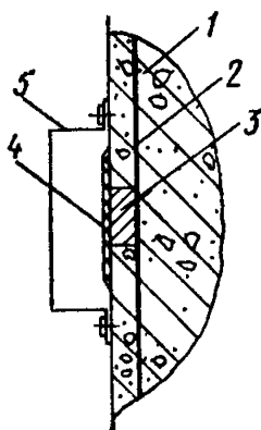
Рис. 12. Пример устройства контрольно-измерительного пункта в надземной железобетонной конструкции 1 — железобетонная конструкция; 2 — арматура; 3 — закладная деталь; 4 — изоляционное покрытие; 5 — коробка из электроизоляционного материала
