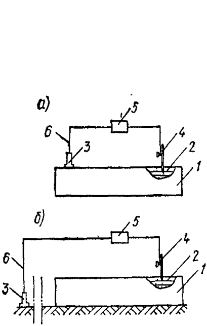
Рис. 19. Схема измерения потенциалов «арматура — бетон» (а) и «арматура — земля» (б)
