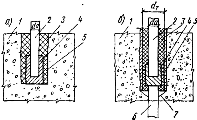
Рис. 33 Примеры обеспечения электроизоляции анкерного стержня в стальной трубе-муфте или в бетоне
