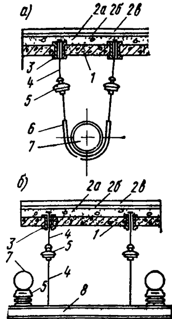
Рис. 15. Пример подвесок типа шпильки для крепления технологических трубопроводов
