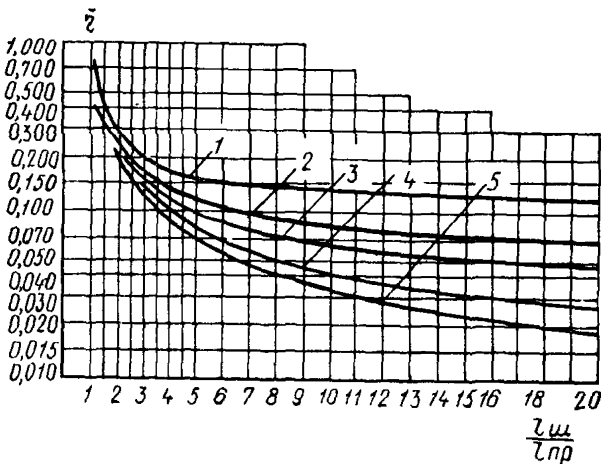
Рис 34. Номограмма для вычисления l_{ш} по \eta и \rho_r 1, 2, 3, 4, 5 — \rho_r соответственно 10, 20, 33, 100 и 200 Ом · м
