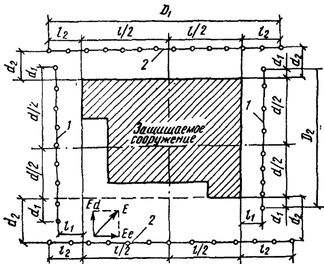
Рис. 35. Пример расположения двух пар заземлений (1 и 2) около сооружения для компенсации блуждающих токов в грунте
