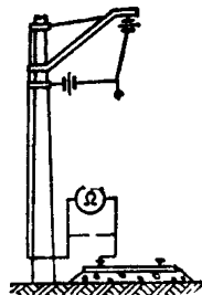
Рис. 21. Схема измерения электрического сопротивления цепи заземления опор при приемке в эксплуатацию
