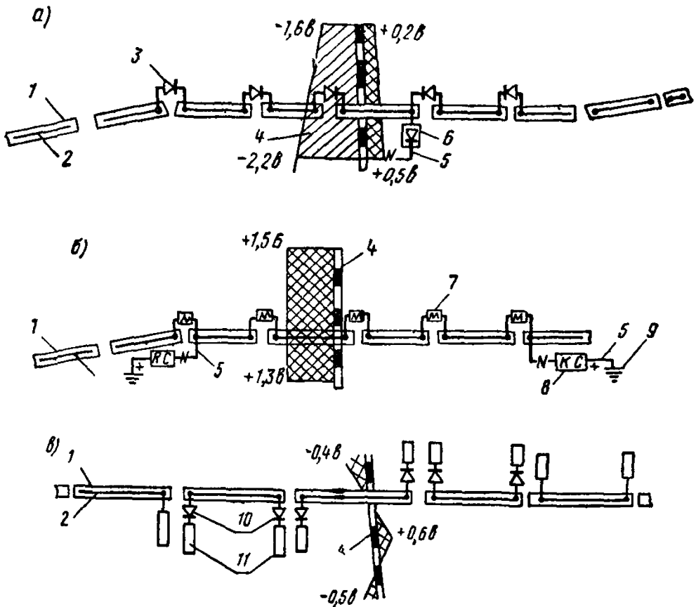
Рис. 39. Схемы защиты блочной железобетонной конструкции
