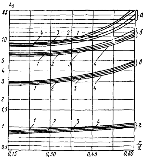
Рис. 30. Номограмма для определения A_2 при h_1/d = 0,0004 - 0,001
