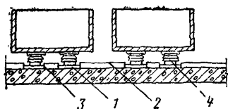
Рис. 9. Закольцовка оснований изоляторов для дренирования токов утечки с изоляторов 1 — металлическое основание изолятора, 2 — металлический соединительный стержень; 3 — сварной стык, 4 — изолятор
