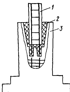
Рис. 32. Пример клеевого соединения железобетонной колонны с фундаментом подванных эстакад
