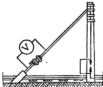
Рис. 26 Схема проверки изоляции анкеров от оттяжек опор контактной сети
