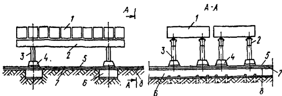
Рис. 4. Пример электроизоляции подванных эстакад отделений электролиза водных растворов от грунтов путем постановки на полы
