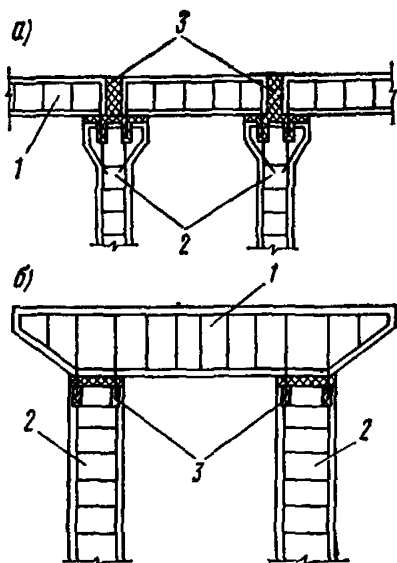
Рис. 31. Примеры клеевых соединений железобетонных конструкций подванных эстакад с разрезкой конструкций
