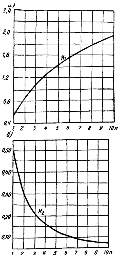
Рис. 4. Графики для определения коэффициентов, необходимых для вычисления кренов фундаментов а — коэффициента k_1 ; б — коэффициента k_2
