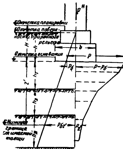
Рис. 1. Расчетная схема распределения давления на горизонтальных сечениях в грунте ниже подошвы фундамента
