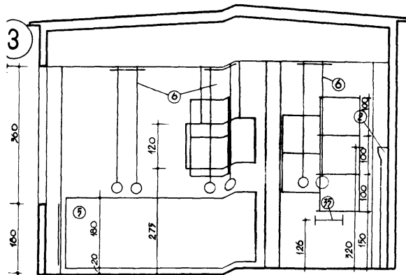
РАЗРЕЗ II-II
