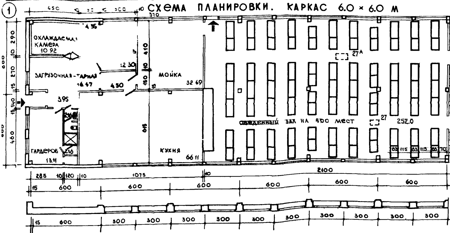
ВАРИАНТ 1 ГАБАРИТНЫЕ СХЕМЫ
