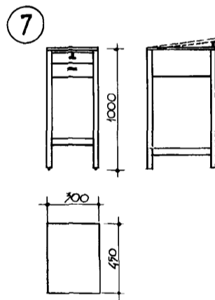
СТОЛ ДЛЯ ПРОЕКЦИОННОЙ АППАРАТУРЫ
