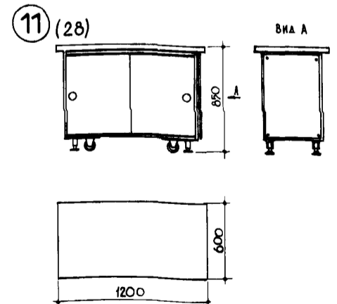
СТОЛ-ВЕРСТАК
