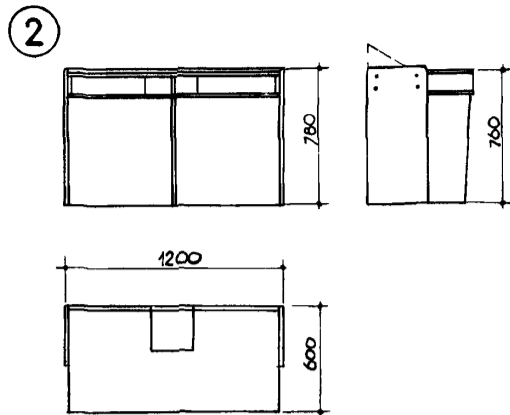
СТОЛ УЧЕНИЧЕСКИЙ ДЛЯ КАБИНЕТА ФИЗИКИ
