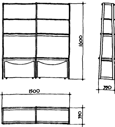
СТЕЛЛАЖ ДЛЯ ТЕРРАРИУМОВ
