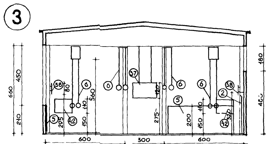
РАЗРЕЗ II-II
