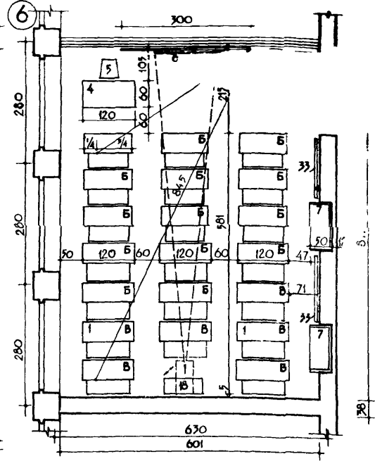
КЛАССНАЯ КОМНАТА ДЛЯ IV КЛАССА С ДВУХМЕСТНЫМИ ПАРТАМИ
