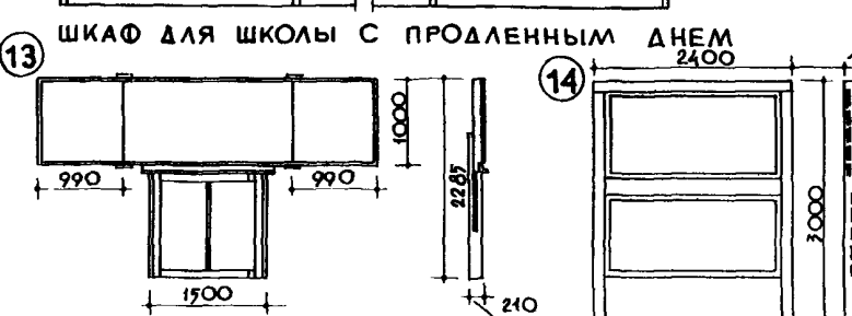
13 ДОСКА РАСКЛАДНАЯ
