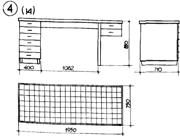
СТОЛ ДЛЯ ЛАБОРАТОРНЫХ ПЕЧЕЙ
