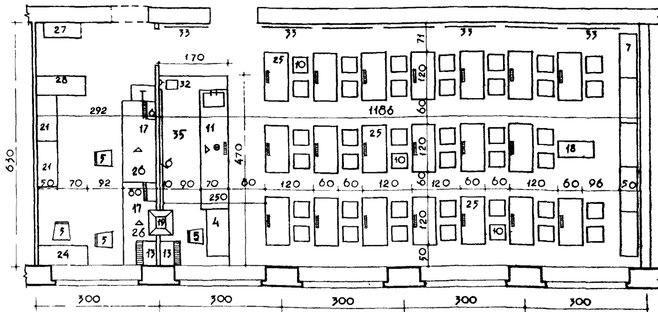
ЛАБОРАТОРИЯ ФИЗИКИ КИРПИЧНЫЕ СТЕНЫ С ШАГОМ 3,00 м
