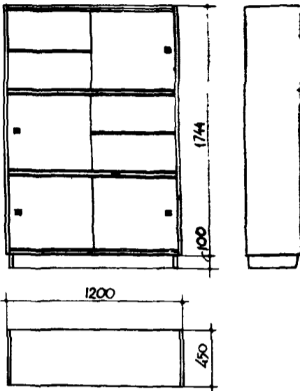
ШКАФ ДЛЯ РЕАКТИВОВ И ПРИБОРОВ
