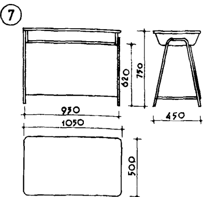
7 СТОЛ УЧИТЕЛЯ НА МЕТАЛЛИЧЕСКОЙ ОСНОВЕ
