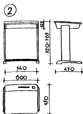
2 СТОЛ ОДНОМЕСТНЫЙ ДЕРЕВЯННЫЙ
