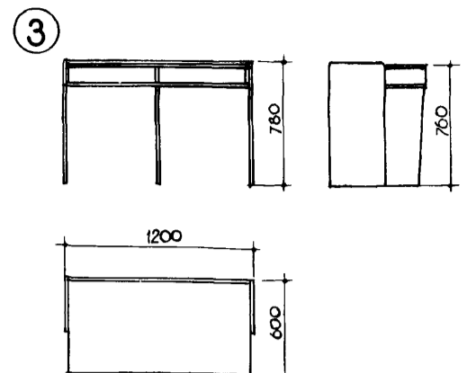
СТОЛ УЧЕНИЧЕСКИЙ ДЛЯ КАБИНЕТА БИОЛОГИИ
