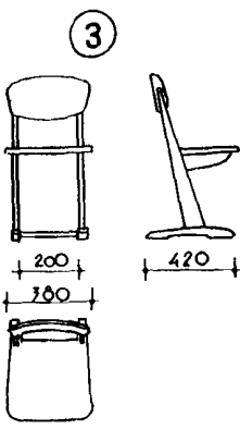
3 СТУЛ ДЕРЕВЯННЫЙ
