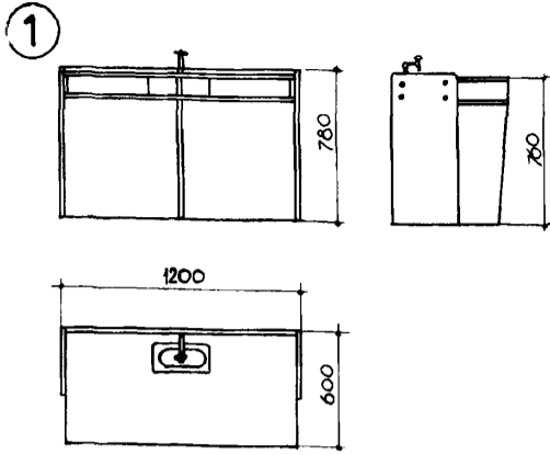
СТОЛ УЧЕНИЧЕСКИЙ ДЛЯ КАБИНЕТА ХИМИИ
