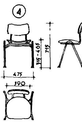
4 СТУЛ НА МЕТАЛЛИЧЕСКОЙ ОСНОВЕ
