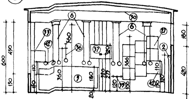
РАЗРЕЗ II-II
