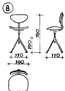
8 СТУЛ УЧИТЕЛЯ НА МЕТАЛЛИЧЕСКОЙ ОСНОВЕ
