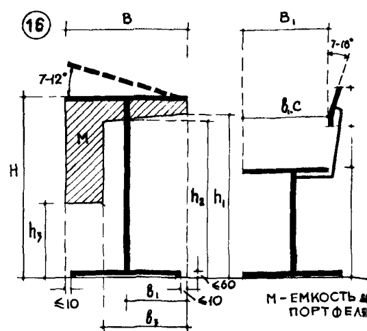
16 ОСНОВНЫЕ РАЗМЕРЫ СТОЛОВ, СТУЛЬЕВ (в мм)
