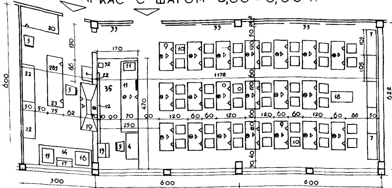
ЛАБОРАТОРИЯ ХИМИИ КАРКАС С ШАГОМ 6,00 x 6,00 м
