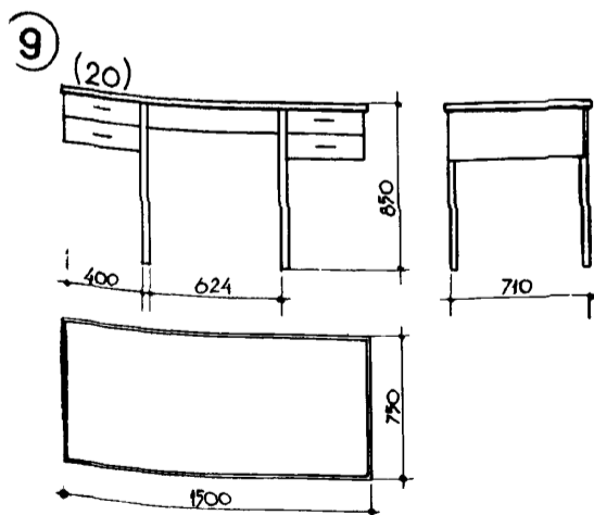
СТОЛ ДЛЯ ПРИБОРОВ
