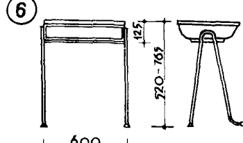
6 СТОЛ ОДНОМЕСТНЫЙ НА МЕТАЛЛИЧЕСКОЙ ОСНОВЕ
