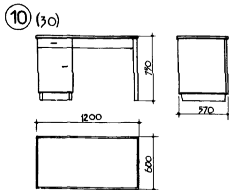
СТОЛ ДЛЯ МИКРОСКОПА
