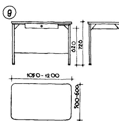
9 СТОЛ УЧИТЕЛЯ ДЕРЕВЯННЫЙ
