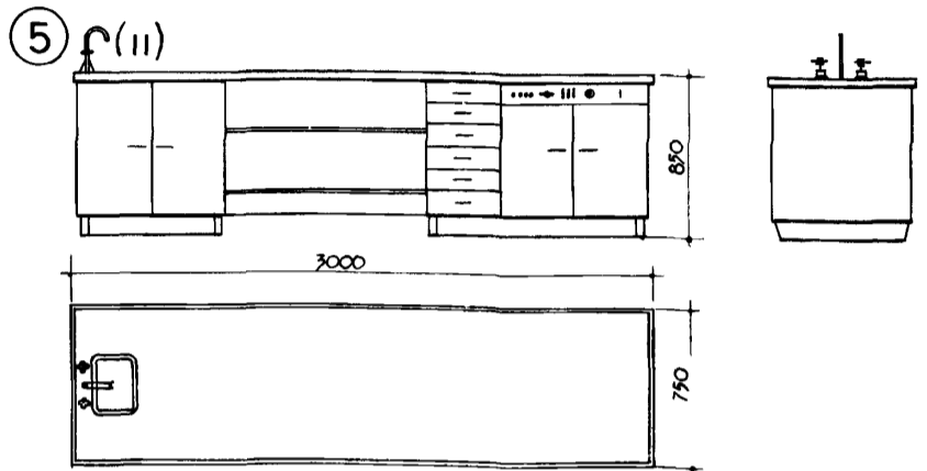
СТОЛ УЧЕНИЧЕСКИЙ ДЛЯ КАБИНЕТА ФИЗИКИ
