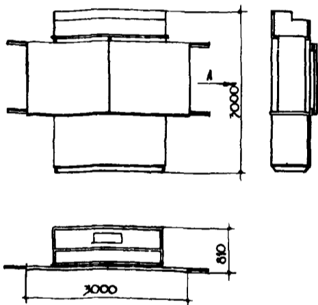
ШКАФ ВЫТЯЖНОЙ/ВСТРОЕННЫЙ/
