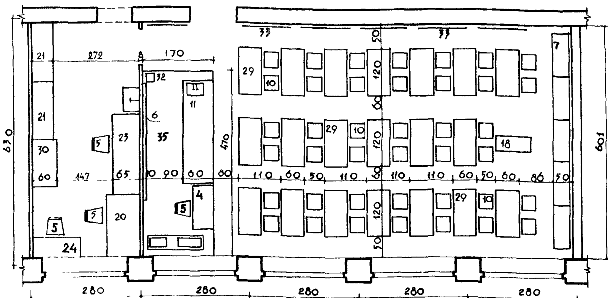
ЛАБОРАТОРИЯ БИОЛОГИИ КИРПИЧНЫЕ СТЕНЫ С ШАГОМ 2,80 м
