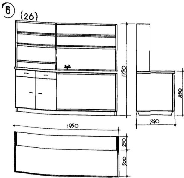
СТОЛ ЛАБОРАТОРНЫЙ ДЛЯ КАБИНЕТА ФИЗИКИ
