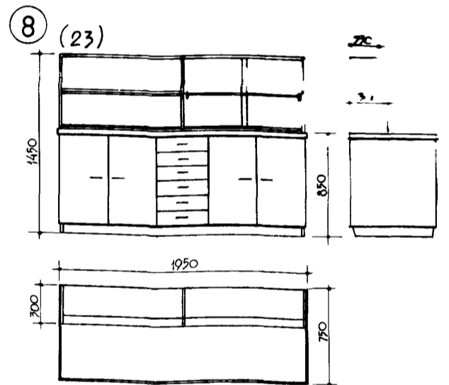
СТОЛ ЛАБОРАТОРНЫЙ ДЛЯ РАБОТЫ С КИСЛОТАМИ
