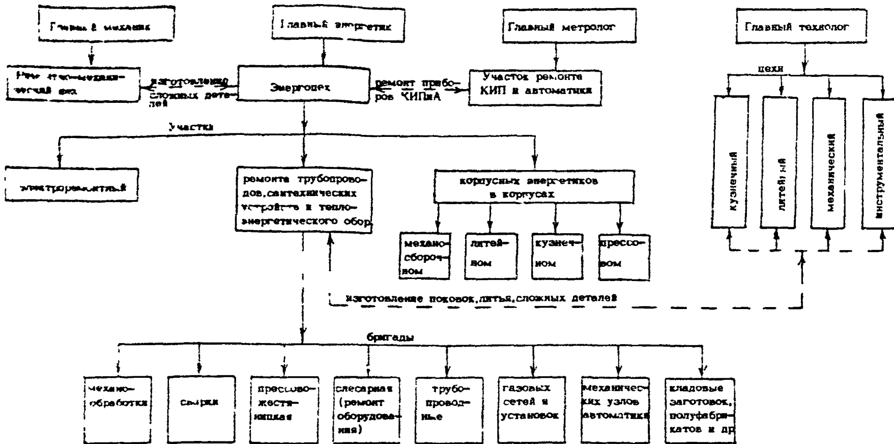
Рис. 2. Организационная схема участка ремонта трубопроводов, санитарно-технических устройств и теплоэнергетического оборудования в энергоцехе предприятия с площадью крытых зданий от 100 до 400 тыс. м 2 .
