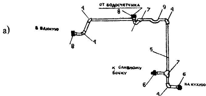
Рис.4. Стояк холодной воды VI в шахт-пакете санузла жилого дома серии КОПЭ:
