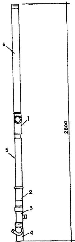
Рис.6. Канализационный стояк в шахт-пакете санузла жилого дома серии КОПЭ:
