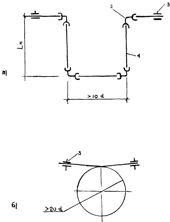
Рис.2. Схемы компенсаторов на водопроводах из полипропиленовых труб:
