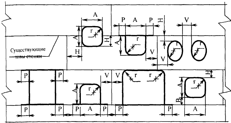
Фиг. 6-1. Приемлемые детали для замены листов стенки
