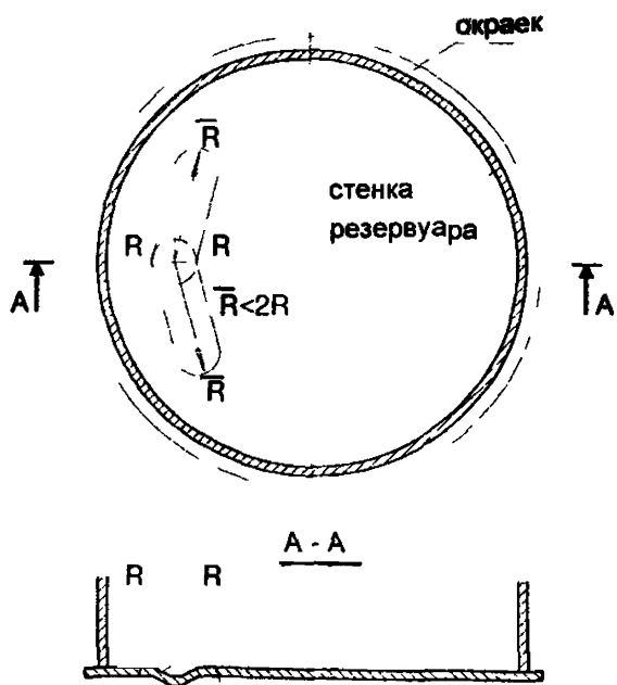
R радиус окружности вписанной в выпучину или впадину f просадка или глубина впадины или выпучины Фиг 5-4 Просадка дна вблизи стенки
