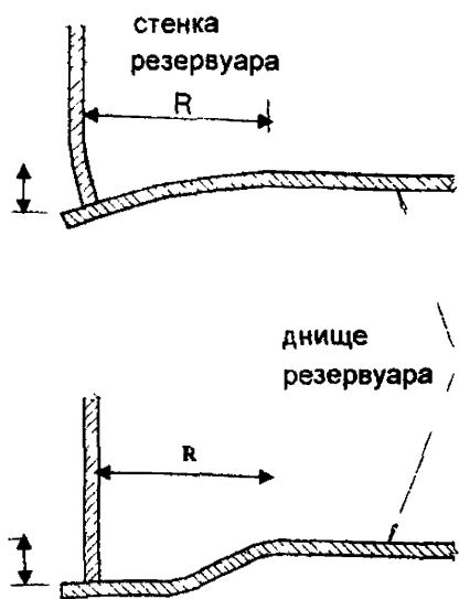
R ширина просадки f глубина просадки Фиг 5-3 Просадка края
