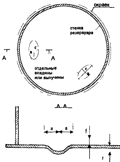
a c малая и большая полуось эллипса описывающего форму выпучины или впадины f глубина впадины или высота выпучины
