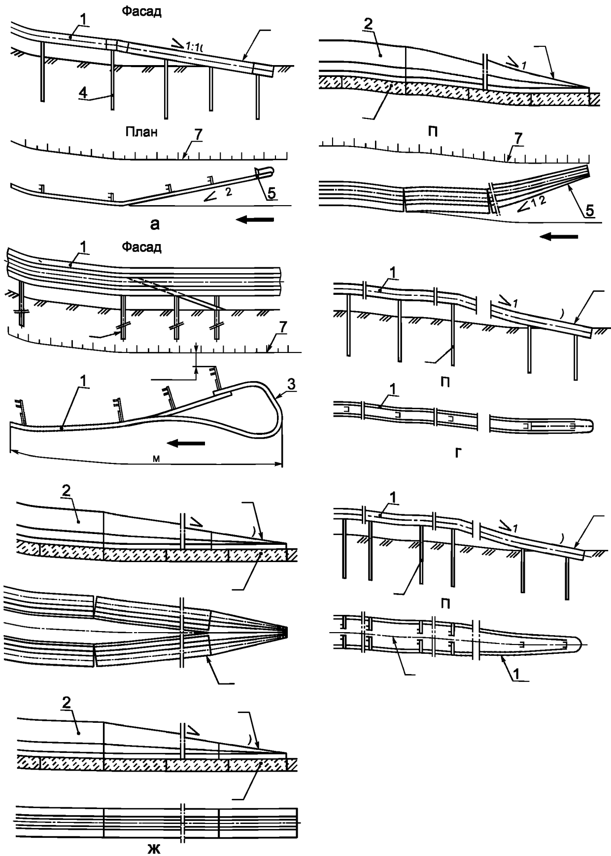
1 — барьерное ограждение; 2 — парапетное ограждение; 3 — изгиб балки ограждения; 4 — стойка ограждения; 5 — отгон ограждения; 6 — понижение ограждения на начальном и конечном участках; 7 — бровка земельного полотна; 8 — основание; 9 — ось разделительной полосы; 10 — сближение рядов ограждения с осью разделительной полосы; ← — направление движения транспортных средств
