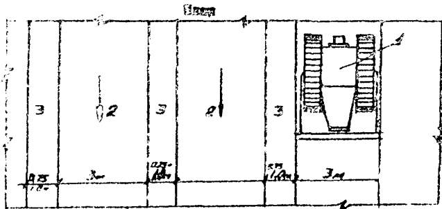
Рис. 2. Срезка растительного слоя: 1 - бульдозер Д-271А; 2 - проходки бульдозера; 3 - промежутки между проходками
