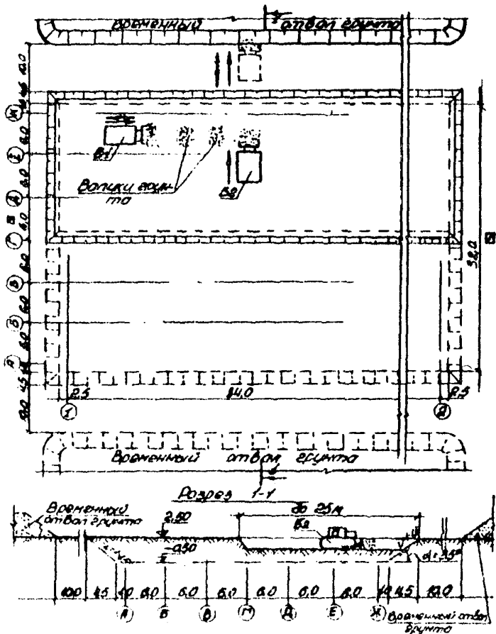
Рис. 1. Схема разработки и перемещения грунта массированным способом:
