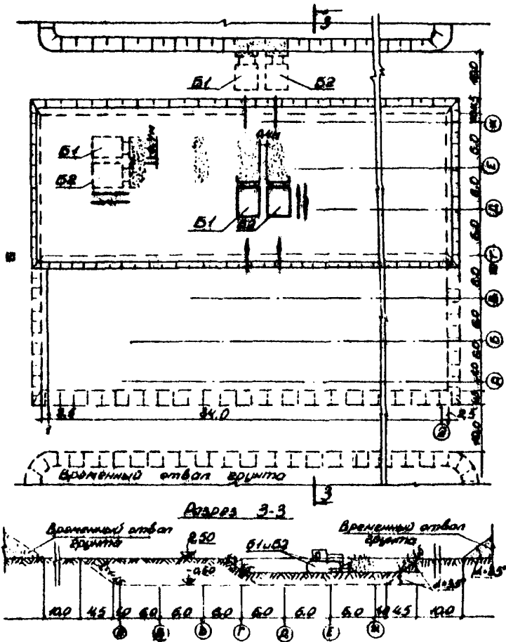
Рис. 3. Схема разработки и перемещения грунта массивным способом:
