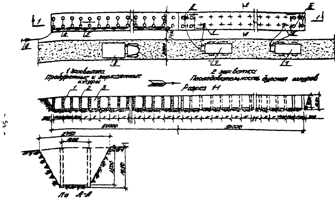
Рис. 2. Схема производства работ: 1 - заряд ВВ; 2 - забочный материал; 3 - взрываема порода; 4 - детонирующий шнур; 5 - протехническое реле КЗДН-58; 6 - электродетонатор; 7 - компрессор ДК-9; 8 - спецмашина на базе автомобиля ГАЗ 52-03; I, II, III, IV - буровые; \rightarrow - общее направление работ; \leftarrow - направление взрыва; \leftarrow - направление бурения
