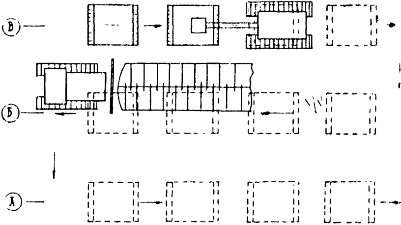
40 40 ① ② ③ ④ СХЕМА ИЗМЕРОВАНИЯ ОТМЕТОК ДНА КОТЛОВАНА
