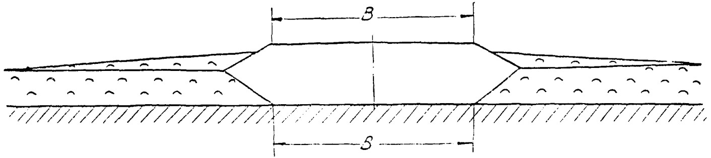
Рис. 22. Насыпь на болотах I и II типов глубиной до 4 м с полным выторфовыванием с укладкой и планировкой вынутаго торфа на откосах
