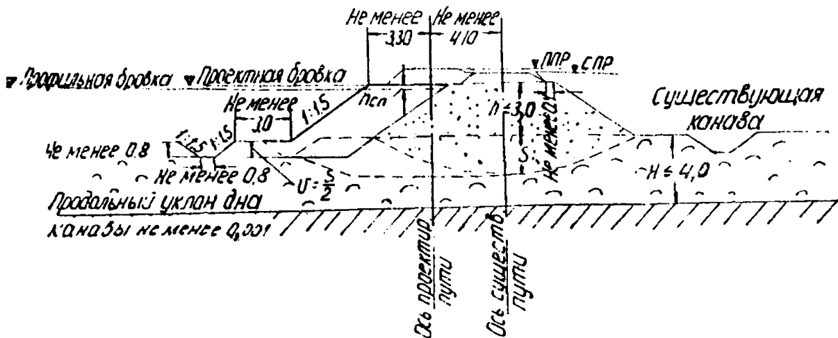
Рис. 13. Насыпь из дренирующих грунтов высотой до 3 м на болотах I типа глубиной до 4 м.
