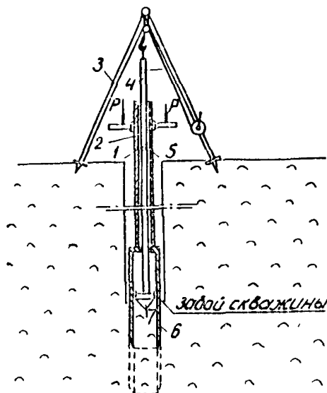
Рис. 5. Схема работы грунтоноса АЛТИ:
