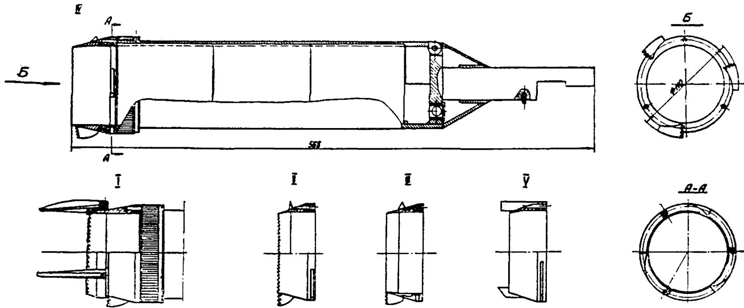
Рис. 4. Универсальный грунтонос конструкции ЦНИИСа для отбора монолитов торфов и других болотных отложений со сменными коронками: I—для слаборазложившихся торфов; II—для хорошо разложившихся торфов; III и IV—для минерализованных торфов и пластичных грунтов; V—для сапрпелей и илов
