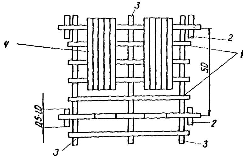
Рис. 29. Земляное полотно на жестком колейном настиле для временных дорог и подъездных путей при однополосном движении:
