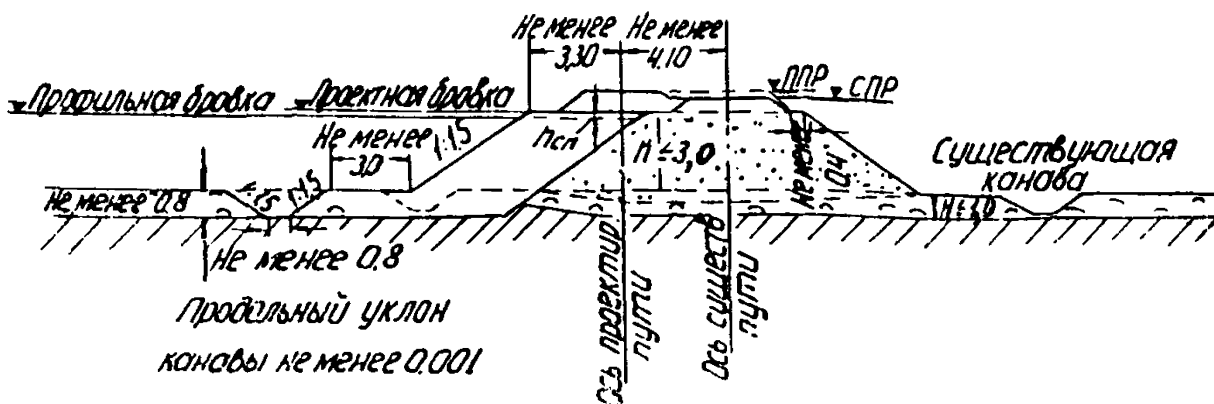
Рис. 12. Насыпь из дренирующих грунтов высотой до 3 м на болотах I типа глубиной до 1 м.
