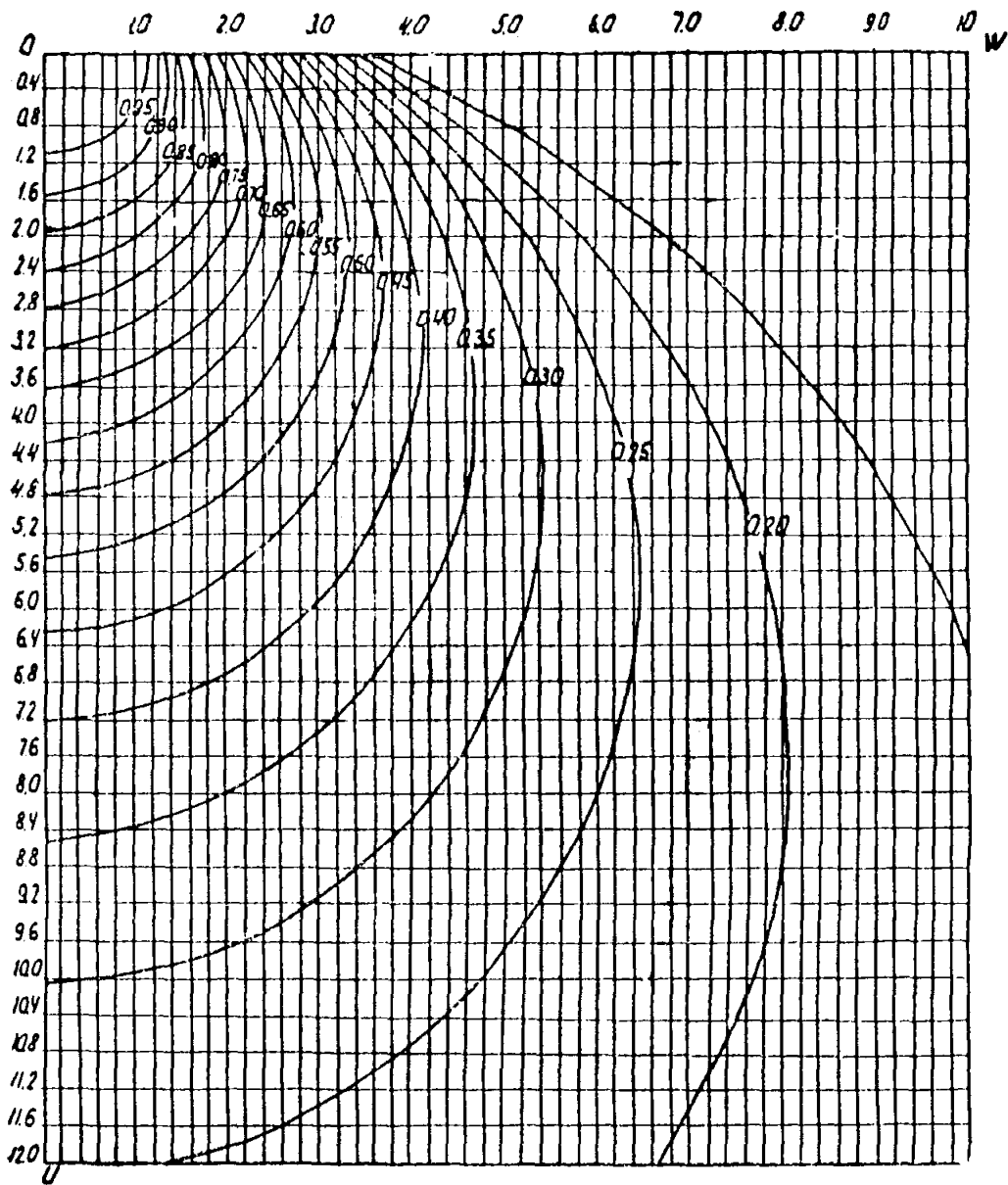
Рис. 5. Графики значений \alpha_1 = \frac{\sigma_1}{\mu_0} при \frac{2a}{B} = 3,0
