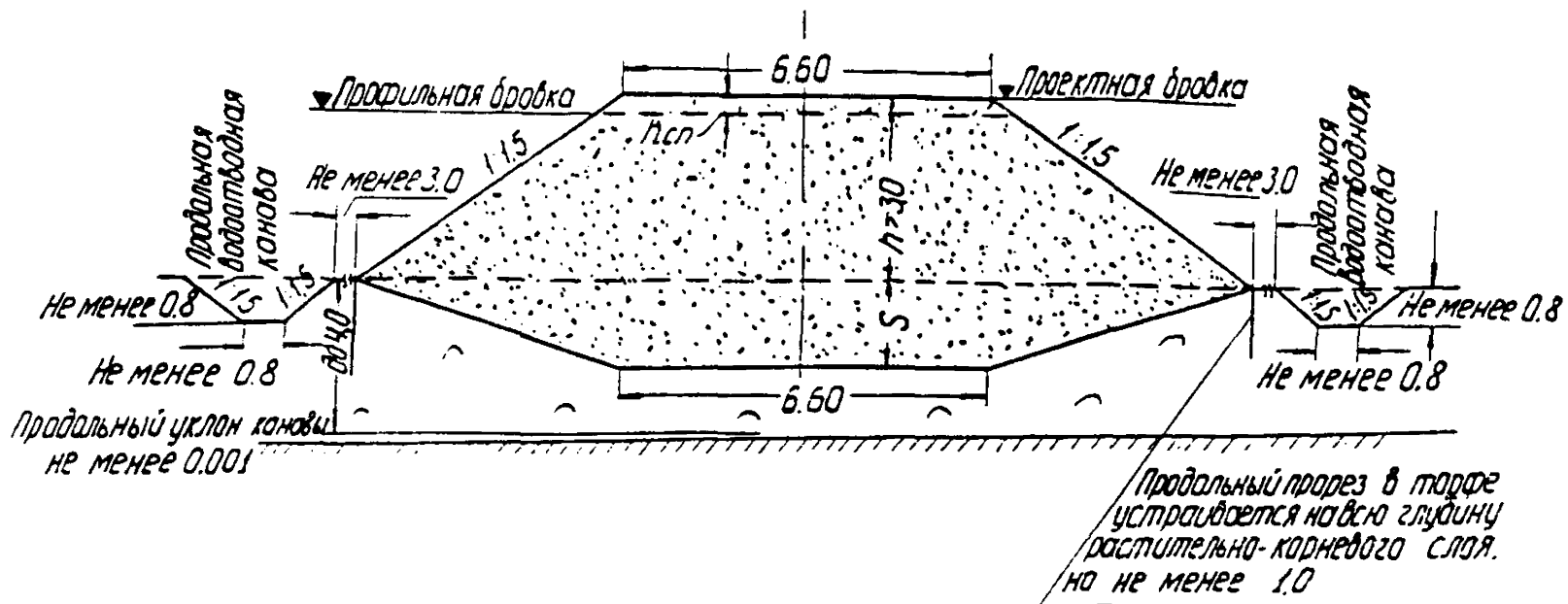
Рис. 8. Насыпь из дренирующего грунта высотой более 3 м на болоте I типа глубиной до 4 м без выторфовывания при поперечном уклоне минерального дна болота не круче 1 : 10 на линиях I и II категорий.
