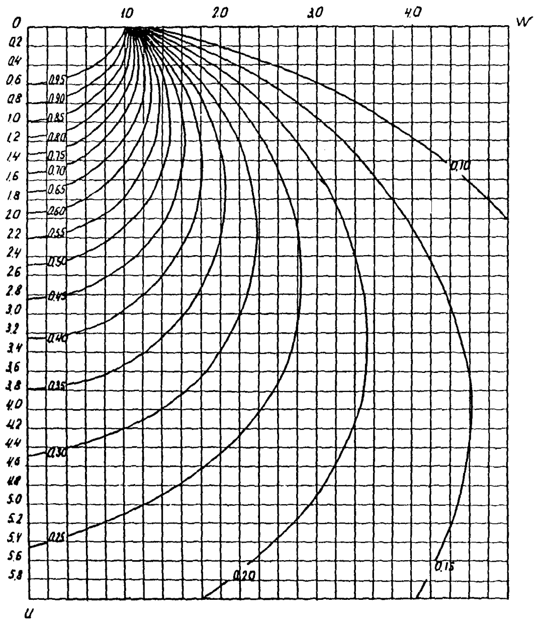
Рис. 2. Графики значений \alpha_1 = \frac{\sigma_1}{\rho_0} при \frac{2a}{B} = 0,2
