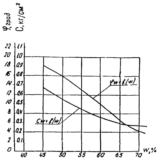
Рис. 7. Зависимость угла внутреннего трения и сцепления от влажности для второго слоя (пл)
