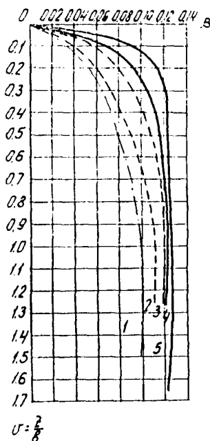
Рис 36. График функции \beta при \varphi = 30^\circ :
