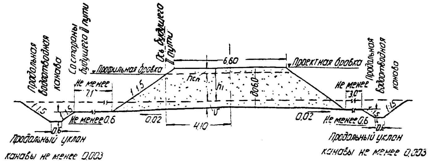
Рис. 16. Насыпь из дренирующих грунтов высотой до 6 м на засоленных грунтах и пухлых солончаках в условиях периодического обводнения основания грунтовыми водами с выходом их на дневную поверхность.
