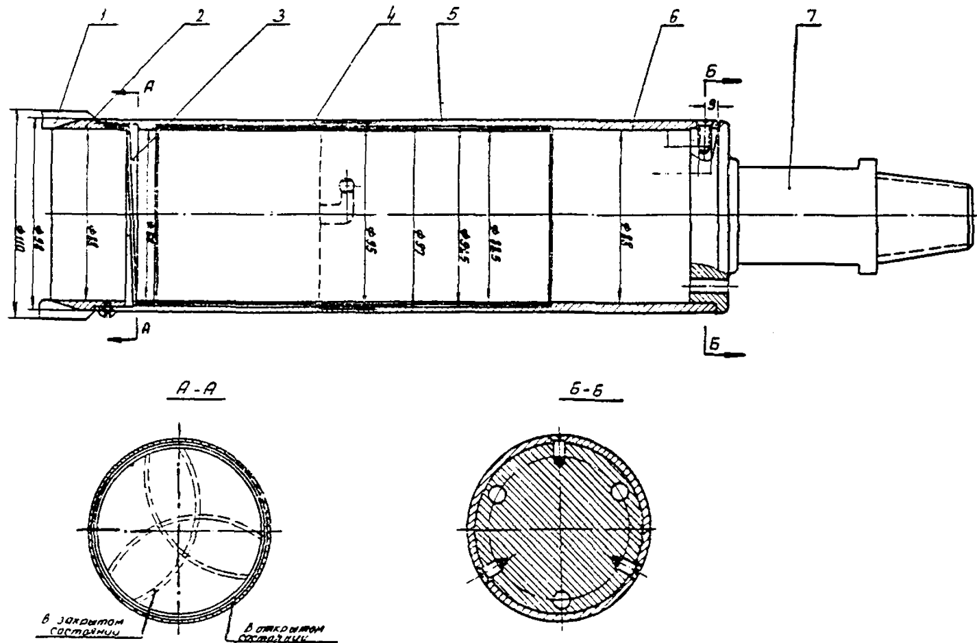
Рис. 3. Грунтонос конструкции Фурса для взятия монолитов илов и других глинистых грунтов мягкопластичной и скрытотекучей консистенции:
