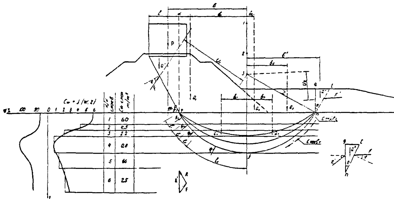
Рис. 37. Расчетная схема для определения устойчивости слабого основания
