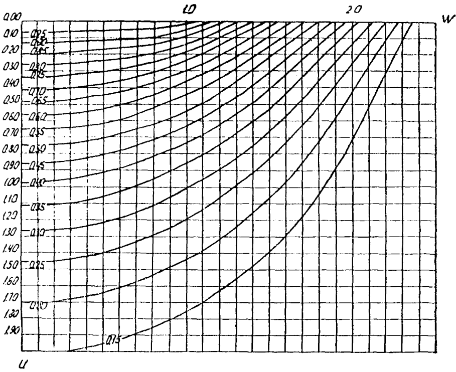
Рис. 12. Графики значений \alpha_2 = \frac{\sigma_2}{\rho_0} при \frac{2a}{B} = 1,6
