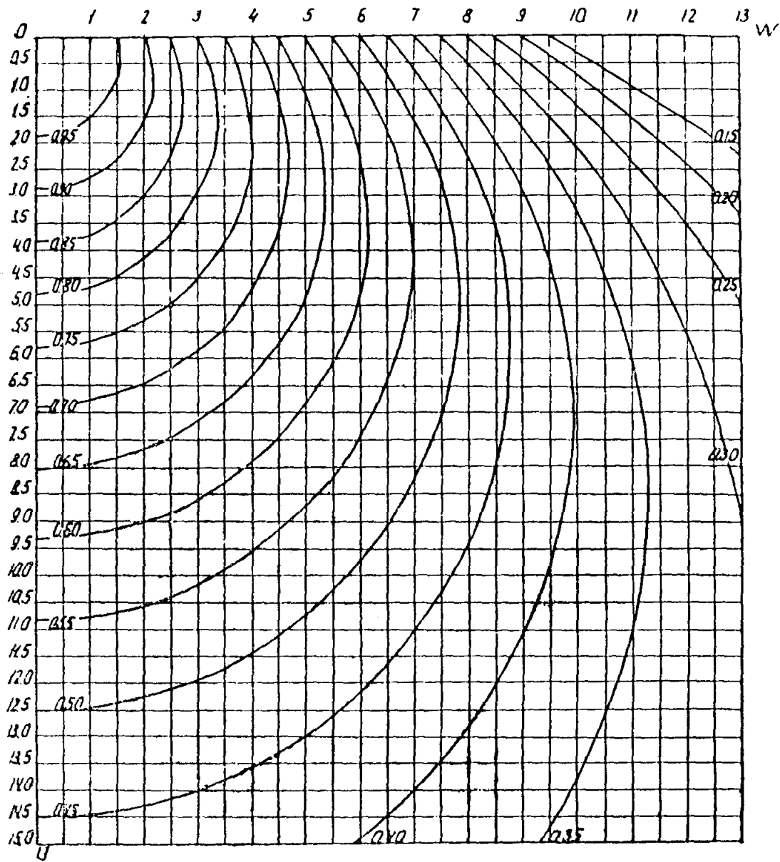
Рис. 7. Графики значений \alpha_1 = \frac{\sigma_1}{p^0} при \frac{2a}{B} = 10
