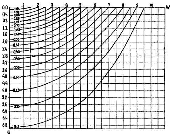
Рис. 15. Графики значений \alpha_2 = \frac{\sigma_2}{\rho_0} при \frac{2a}{B} = 10
