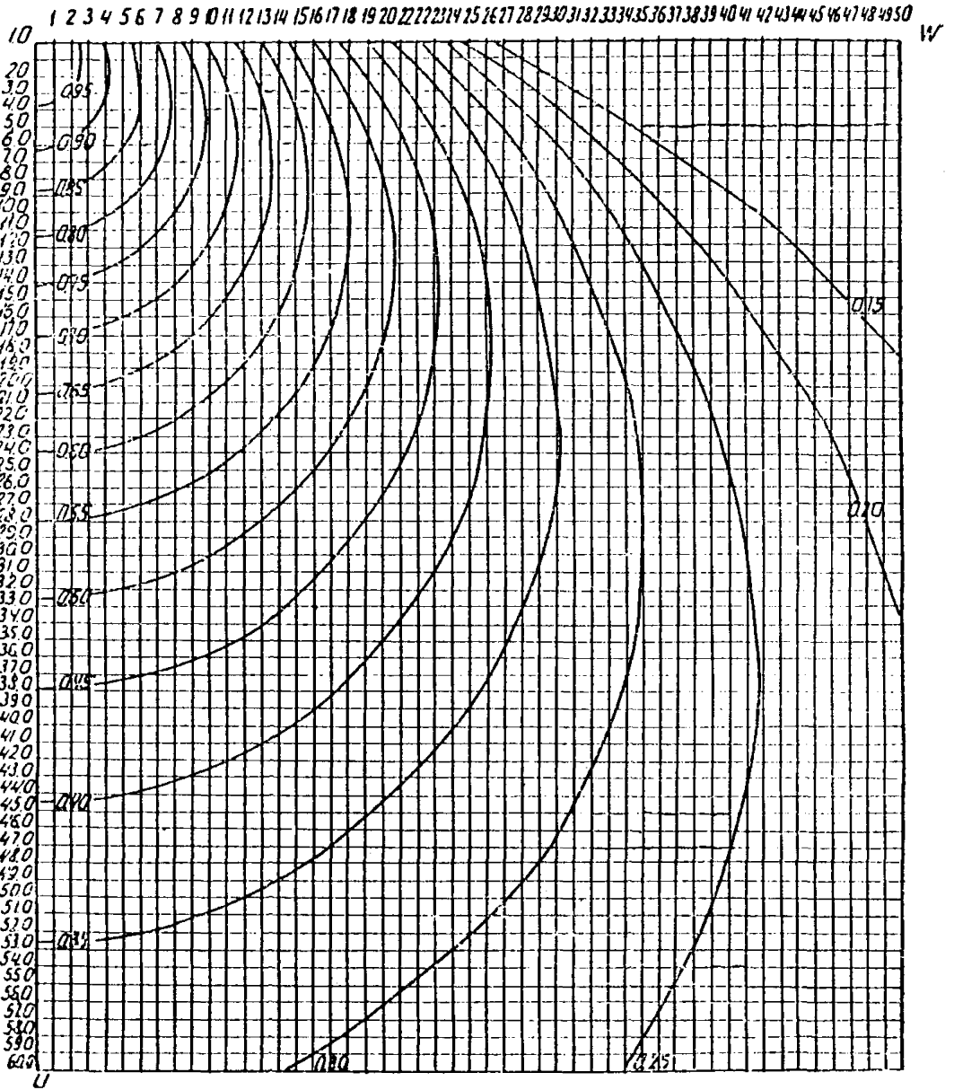
Рис. 8. Графики значений \alpha_1 = \frac{\sigma_1}{\rho_0} при \frac{2a}{B} = 30
