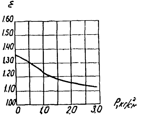
Рис. 3. Компрессионная кривая глины текучепластичной консистенции
