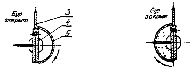
Рис. 1. Торфяной бур ТБ-5: 1—винт; 2—полуконус; 3—нож; 4—сердечник; 5—ложка
