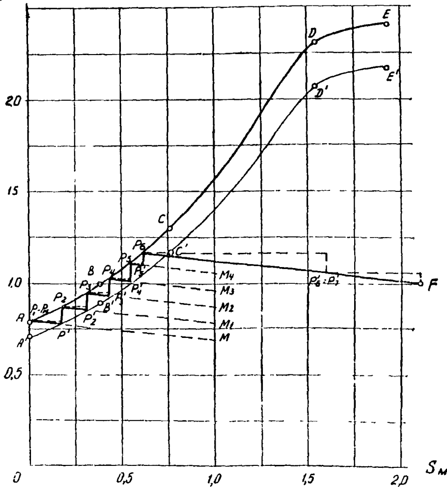
Рис. 8. Определение ступеней нагрузки при наиболее рациональном режиме отсыпки насыпи
