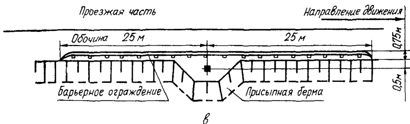
Рис. 5. Установка ограждений:
