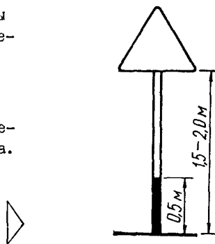
Рис. 8. Рекомендуемая окраска опор дорожных знаков
