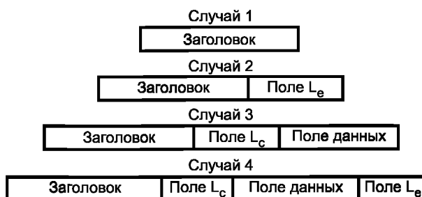
Рисунок 4 — Четыре структуры командных APDU
