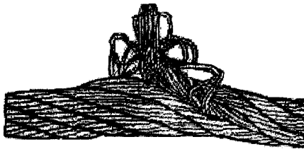
Рис. 11. Выдавливание сердечника
