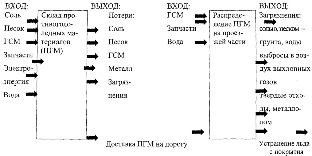
Рис.1. Принципиальная поэтапная схема операций борьбы с гололедом
