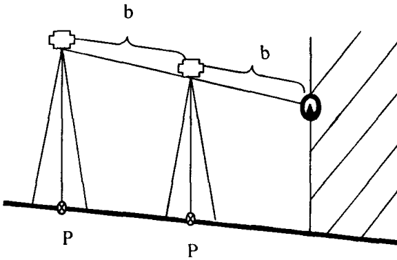
Рис.5. Схема разбивки по высоте створа для установки вспомогательных точек.
