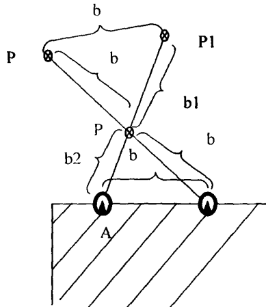
Рис.4. Схема определения пространственных координат стенных пунктов наземной сети по спутниковым наблюдениям на вспомогательных точках двух створов.
