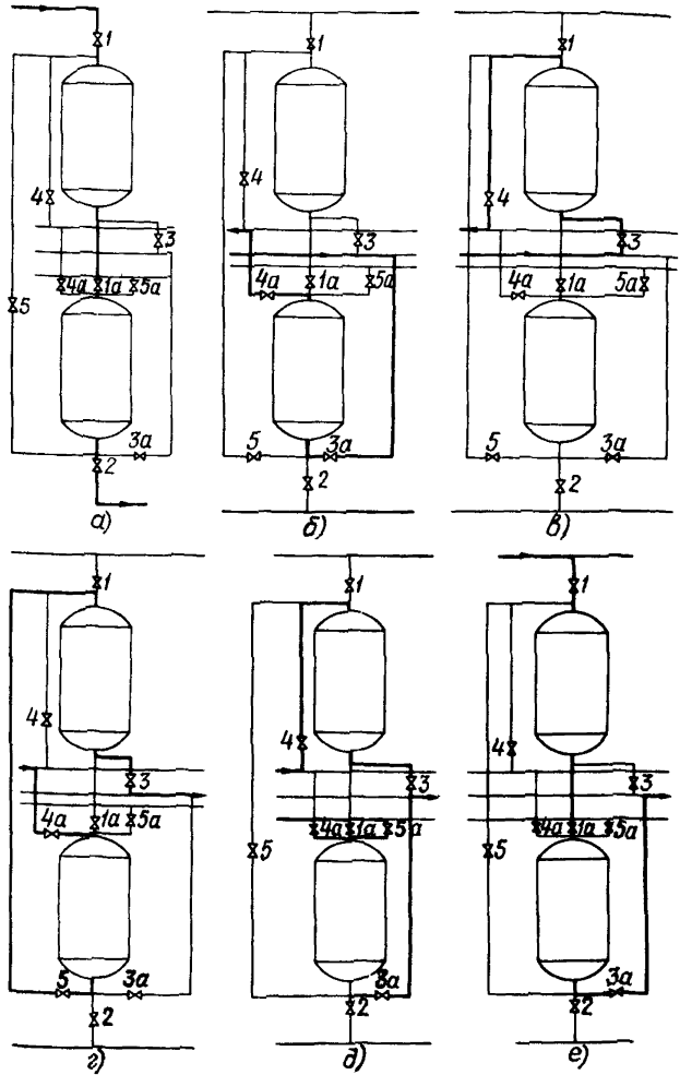
Рис. 6-4. Схема потоков воды при различных стадиях эксплуатации ступенчато-противоточного ионитового фильтра: а - фильтрование; б - взрыхление второго корпуса; в - взрыхление первого корпуса; г - регенерация; д - раздельная отмывка первого корпуса и доотмывка второго корпуса; е - последовательная отмывка первого и второго корпусов 1-5; 1а, 3а - 5а - задвижки
