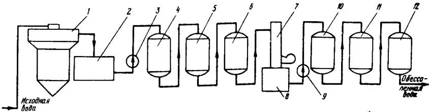
Рис. I-1. Схема обработки воды методом трехступенчатого обессоливания:
