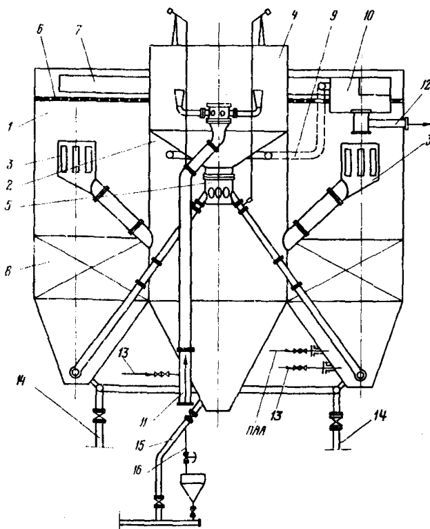
Рис.2-2. Схема осветлителя ВТИ производительностью 350 м 3 /ч
