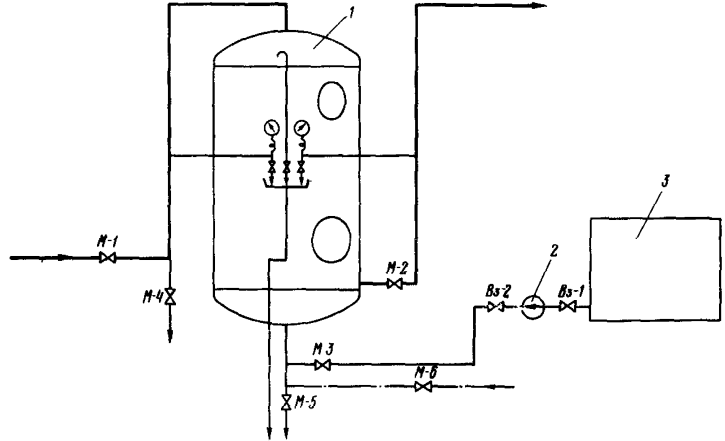
Рис.4-2. Схема обслуживания однокамерного механического фильтра:
