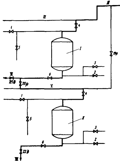
Рис.6-5. Схема последовательной регенерации фильтров:
