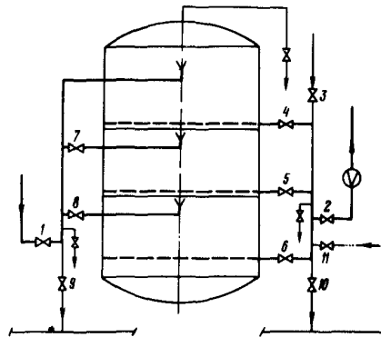
Рис. 4-4. Схема обслуживания трехкамерного механического фильтра
