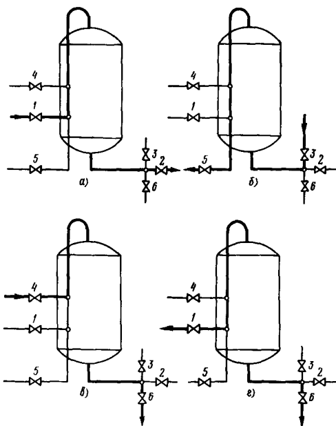
Рис.6-1. Схема потоков воды при различных стадиях эксплуатации прямоочного ионитового фильтра:
