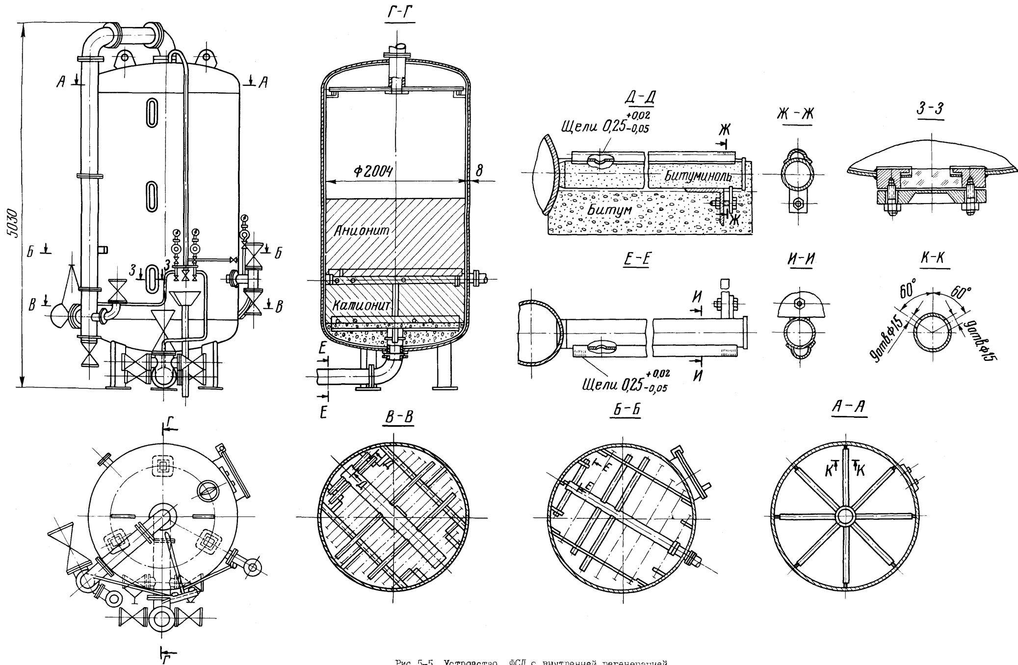
Рис. 5-5. Устройство ФСД с внутренней регенерацией
