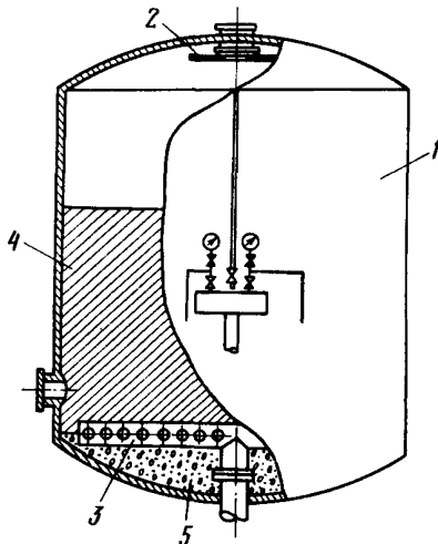
Рис.4-1. Устройство вертикального однокамерного механического фильтра
