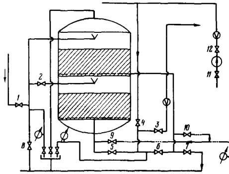
Рис. 4-3. Схема обслуживания двухкамерного механического фильтра
