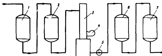
Рис.5-1. Схема глубокого химического обессоливания воды:
