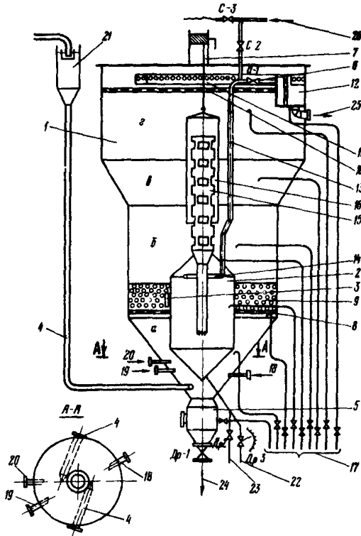
Рис.3-1. Схема осветлителя СНИИ-I производительностью 200 м 3 /ч:
