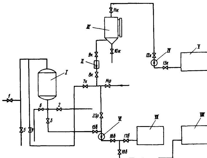
Рис.6-2. Схема регенерации ионитового фильтра с насосами-дозаторами крепкого реагента:
