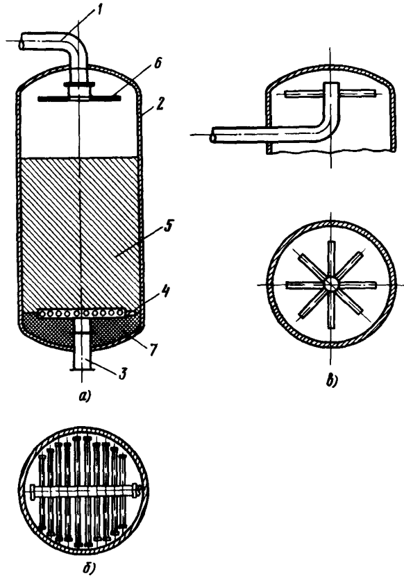
Рис.5-3. Устройство прямоточного мониторингового фильтра:
