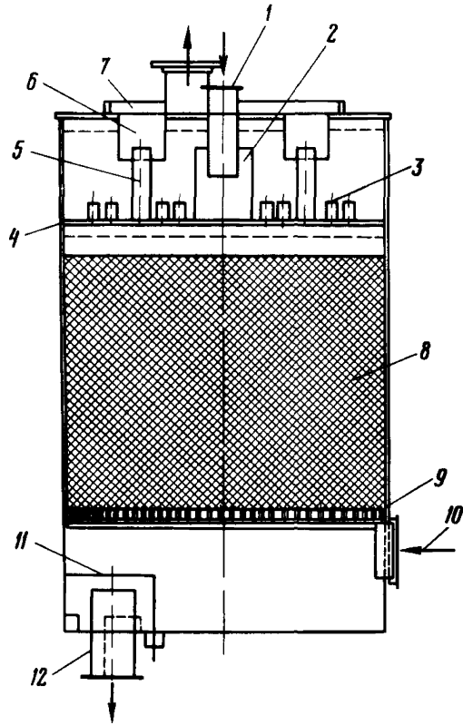
Рис.5-2. Общий вид декарбонизатора
