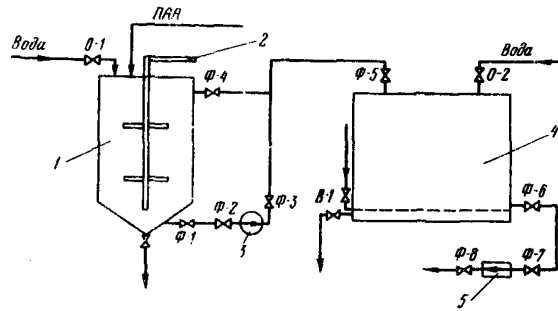
Рис.2-4. Схема приготовления и дозирования ППА
