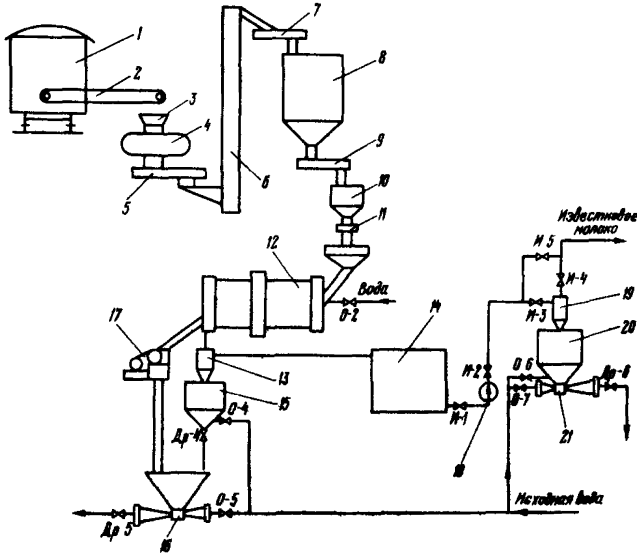
Рис. 3-3. Схема разгрузки и хранения извести
