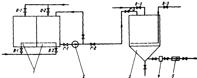
Рис.2-3. Схема приготовления и дозирования коагулянта - сернистого алюминия
