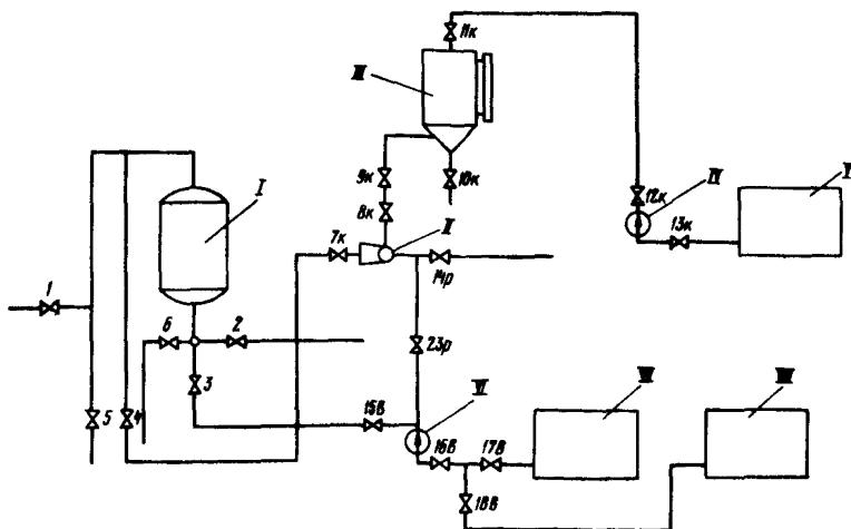
Рис.6-6. Схема подачи на фильтр реагента с помощью гидроэлеватора:
