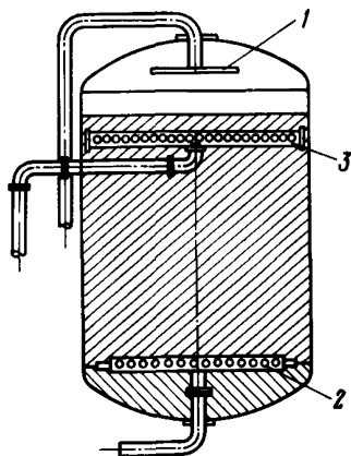
Рис.5-4. Устройство противоточного монитового фильтра: 1-3 - соответственно верхнее нижнее и среднее дренажно-распределительное устройство
