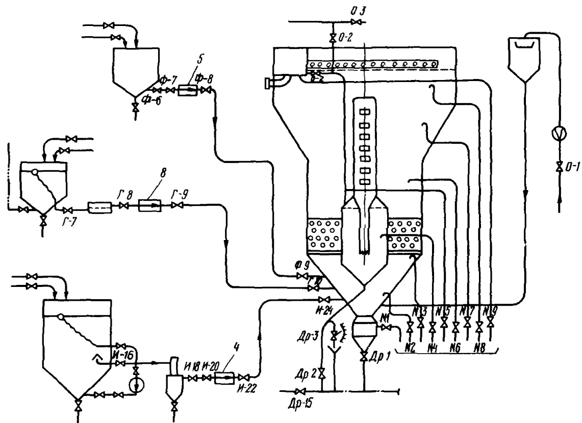
Рис.3-6. Схема обслуживания осветителя для известкования
