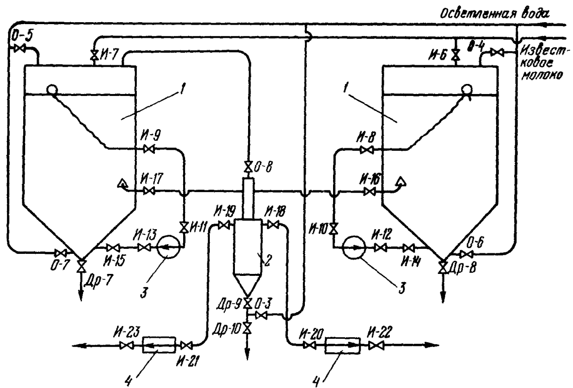
Рис.3-4. Схема приготовления и дозирования известкового молока
