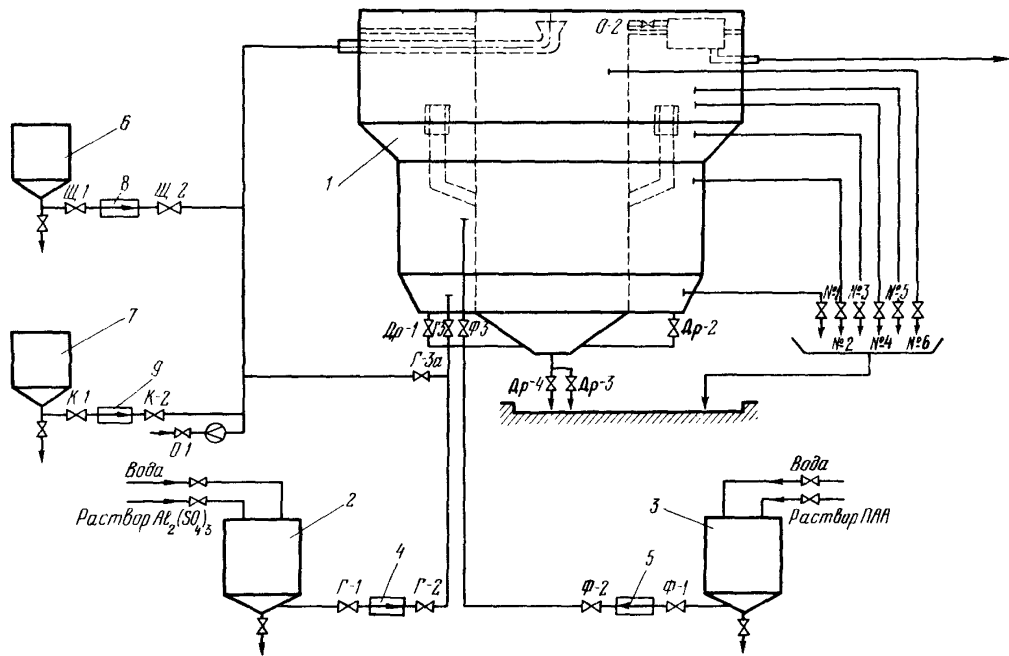
Рис.2-5. Схема обслуживания осветителя для коагуляции
