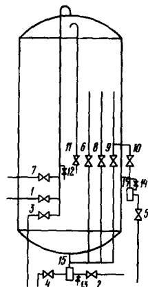
Рис.6-7. Схема наружных трубопроводов ФСД с внутренней регенерацией
