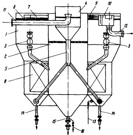
Рис.2-1. Схема осветлителя ЦНИИ-2 производительностью 450 м 3 /ч
