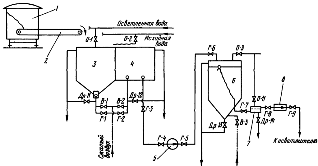
Рис.3-5. Схема приготовления и дозирования коагулянта (серножелезистого железа)
