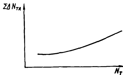
Рис. 16. Зависимость суммарных потерь турбоагрегата от электрической мощности
