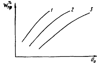
Рис.18. Зависимость удельной выработки электроэнергии на тепловом потреблении от расхода свежего пара при постоянных \rho_{ртв} (линии 1,2,3)
