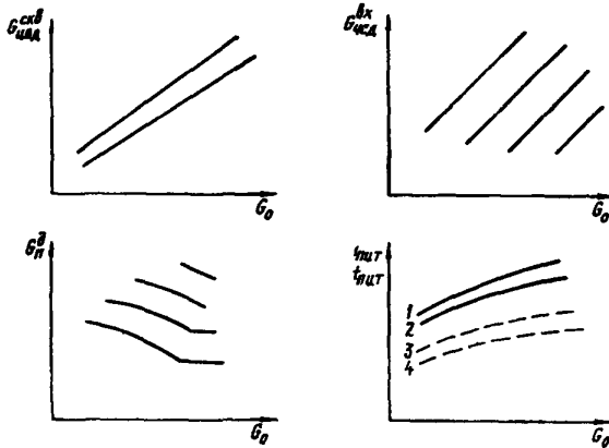
Рис.31. Зависимости расходов пара через ЦВД (при p_{п} = const ), на входе в ЧСД (при G_{п} = const ) и в деаэратор (при G_{п} = const ), а также конечной температуры и энтальпии питательной воды от расхода свежего пара:
