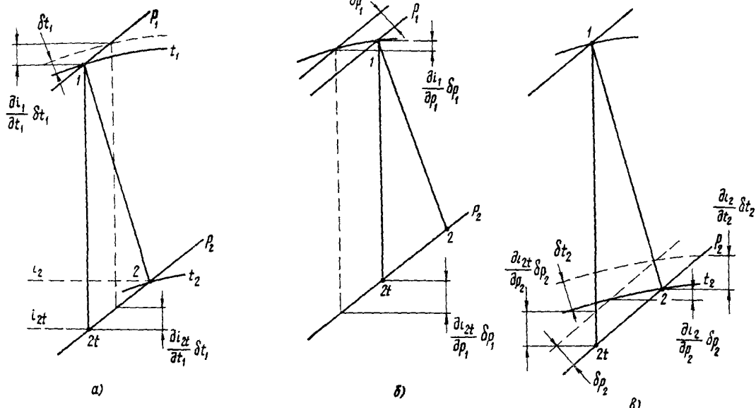
Рис. П.2. Влияние погрешностей измерения температур t_1, t_2 и давлений p_1, p_2 на значение использованного и располагаемого теплоперепадов: а - влияние t_1 ; б - влияние p_1 ; в - влияние p_2 и t_2
