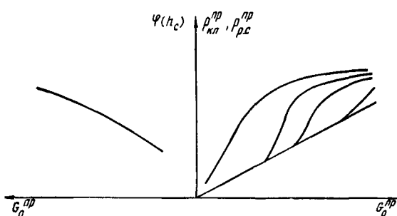
Рис.37. Зависимость давления за регулируемыми клапанами ( \rho_{кл}^{np} ) в камере регулирующей ступени ( \rho_{rc}^{np} ) и угла поворота кулачкового вала ( \psi ) или подъема поршня сервомотора от расхода свежего пара ( G_o^{np} ) при номинальных параметрах
