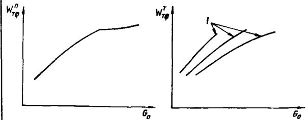
Рис.36. Зависимости удельной выработки электроэнергии на тепловом потреблении от расхода свежего пара: 1 - Q_n = \text{const}
