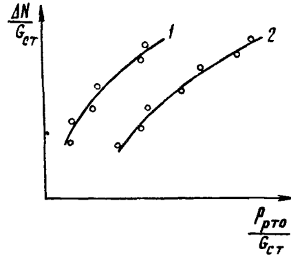
Рис.8. "Универсальные" кривые поправки к мощности на изменение давления пара в РГО:
