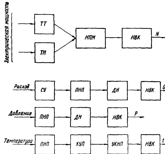
Рис. П. I. Схемы каналов измерения основных технологических параметров:
