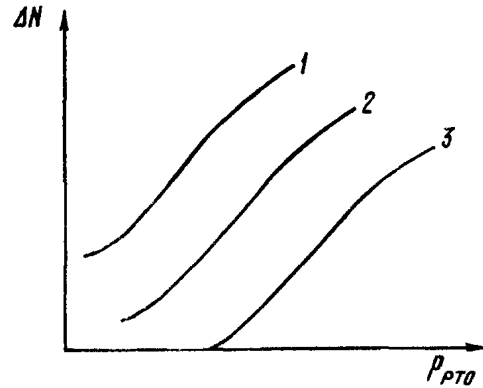
Рис.9. Сетка поправок к мощности на изменение давления пара в РГО при постоянных расходах через ступень, предшествующую РГО:
