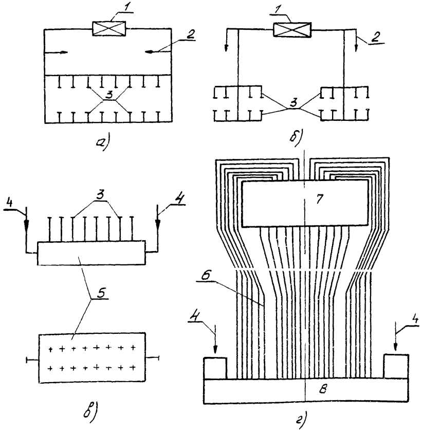
Рис. 1. Схемы распределения вторичного (а, б, г) и первичного (д) воздуха по горелкам:
