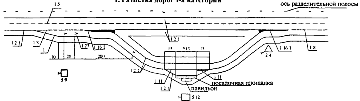
Остановка с пешеходным переходом в разных уровнях
