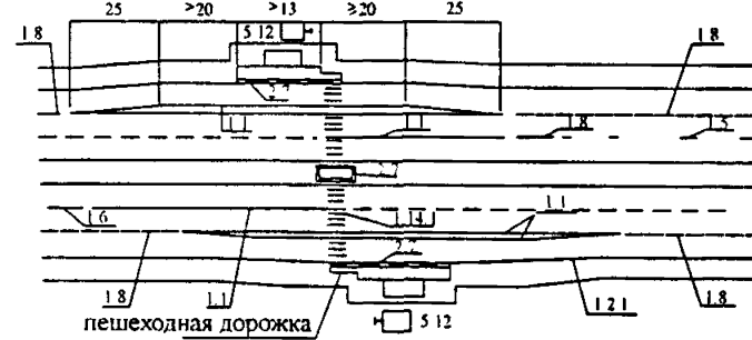
Остановка с пешеходным переходом в одном уровне
