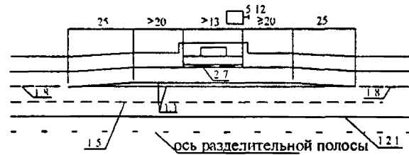
Остановка в зоне примыкания дороги
