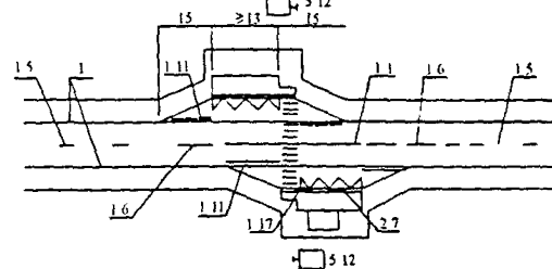
4. Разметка дорог IV категории при отсутствии переходно-скоростных полос
