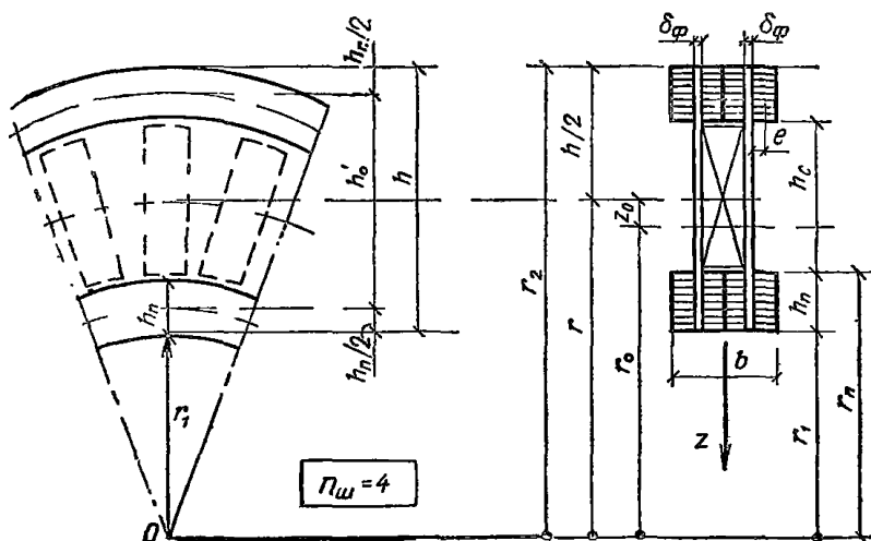
Рис. 9. Геометрические характеристики гнутосклеенного элемента с фанерными стенками
