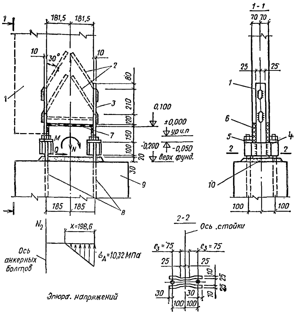
Рис. 58. Опорный узел рамы
