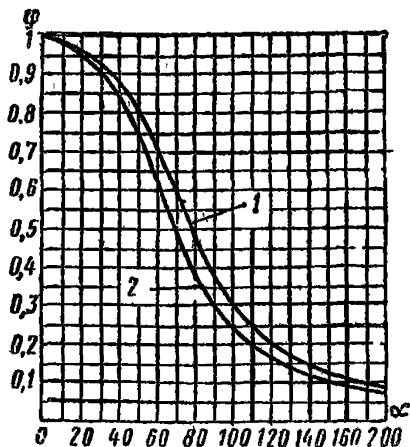
Рис. 70. График определения коэффициента продольного изгиба \varphi по формулам (7) и (8) СНиП 11-25-80
