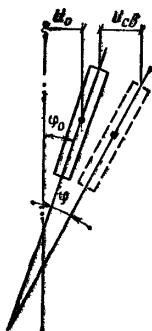
Рис. 64. Перемещение поворота и погни дощатоклееной балки покрытия из ее плоскости в середине пролета, выполняющей функцию пояса поперечной связевой фермы
