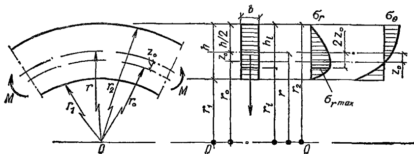
Рис. 8. Геометрические характеристики и эпюры радиальных и тангенциальных нормальных напряжений гнутосклеенного элемента
