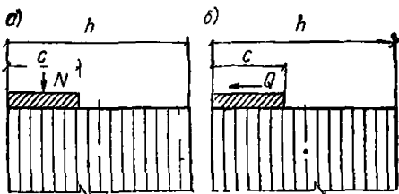
Рис. 20. Схема загрузки конца деревянного элемента местной нагрузкой а) вдоль волокон; б) поперек волокон
