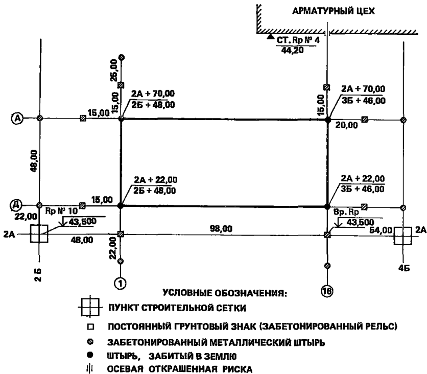
Рис. 14. Схема закрепления и привязки основных осей здания
