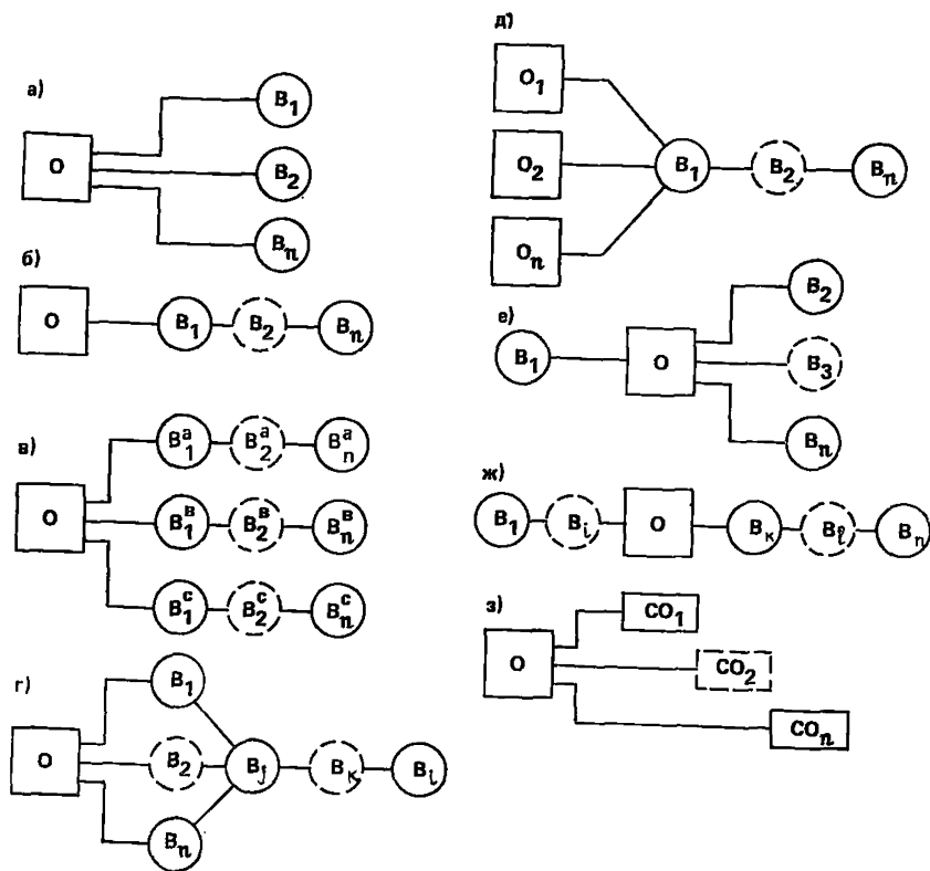
Рис. 3. Характерные виды схем комплексной механизации а — основное (ведущее) монтажное средство O и несколько параллельно работающих вспомогательных (комплектующих) монтажных средств B ; б — то же, последовательно, в—ж — то же, комбинированно; з — основное монтажное средство с комплектом сменного рабочего оборудования CO
