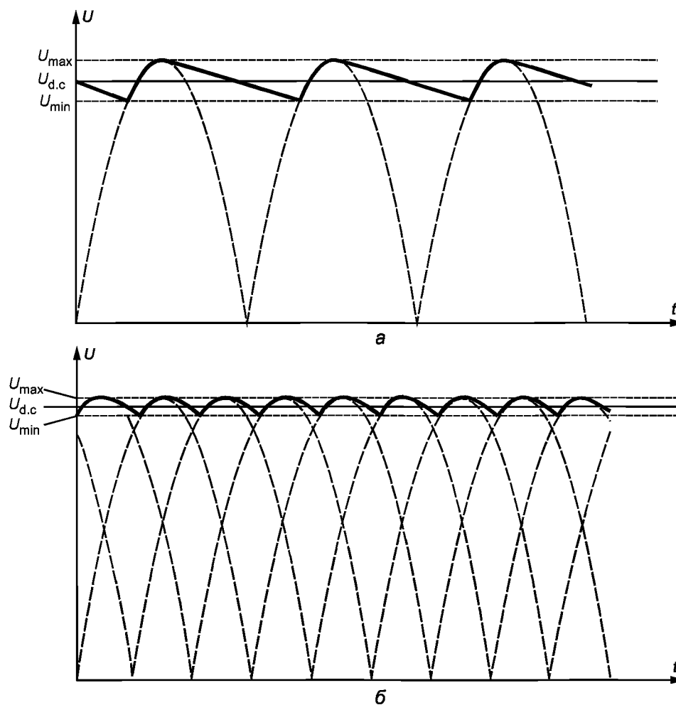
a — однофазный выпрямитель; б — трехфазный выпрямитель
