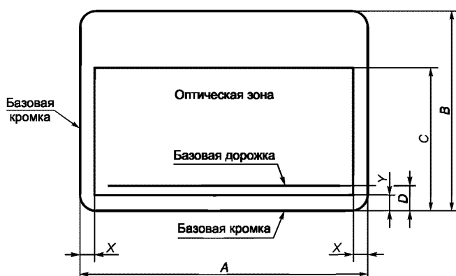
Рисунок 1 — Размеры и расположение оптической зоны
