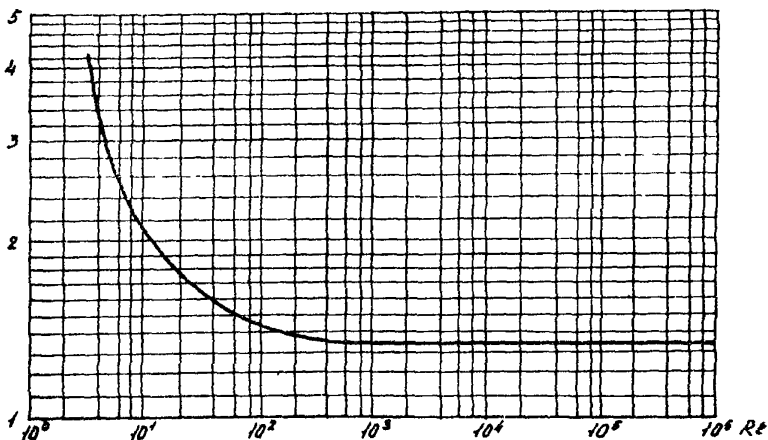
Рис. 1. График определения коэффициента K функции от числа Рейнольдса
