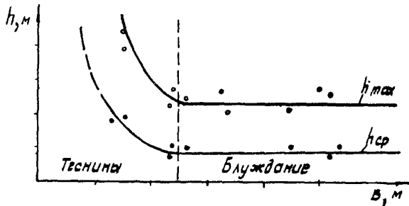
Рис. 6. График средних глубин блуждающей реки
