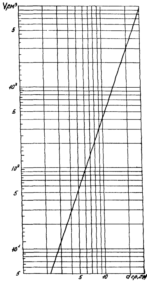
Рис.2П. Зависимость объема V от среднего диаметра d_{\text{cp}}
