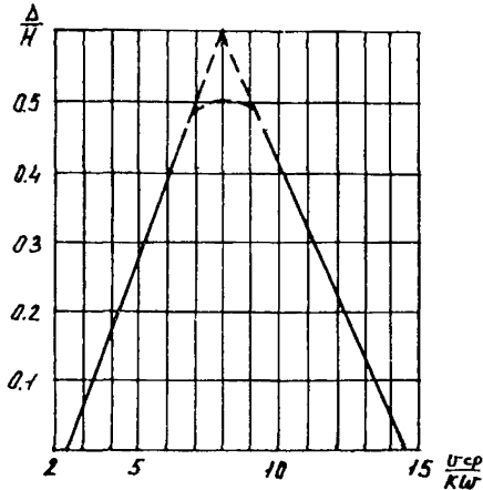
Рис.5. Зависимость относительной высоты гряды \frac{\Delta}{H} от критерия \xi = \frac{v_{cp}}{Kw}
