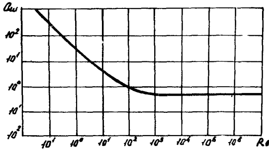
Рис. 2. Коэффициент сопротивления шара в функции числа Рейнольдса сопротивлений и соответствует Re > 2400 . Такой режим наблюдается при обтекании естественных частиц крупнее 3-5 мм.
