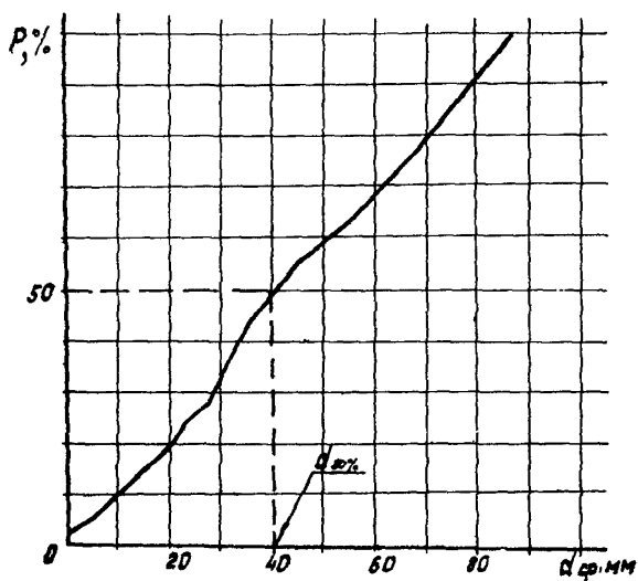
Рис. 3П. Интегральная кривая распределения гранулометрического состава
