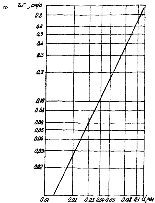
Рис.3. График для определения гидравлической крупности частиц песка
