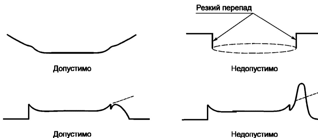
Рисунок 4 — Примеры профилей поверхности
