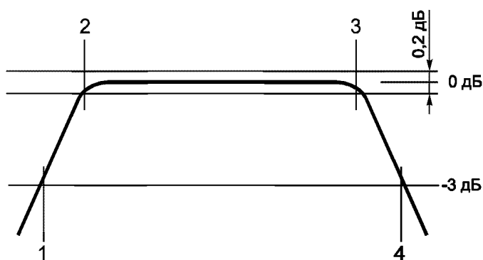
Рисунок Б.1 — Характеристики полосового фильтра
