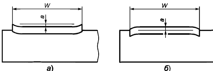
Рисунок 3 — Профиль поверхности
