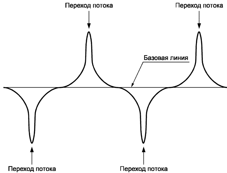
Рисунок 7 — Пример формы сигнала
