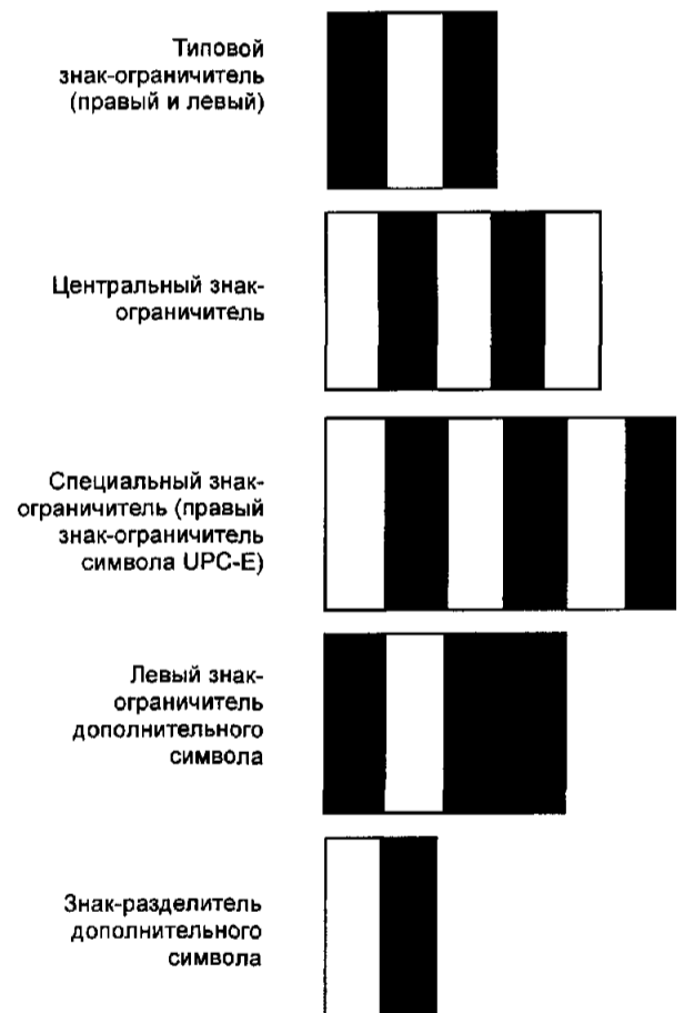
Рисунок D.2 — Представление вспомогательных знаков
