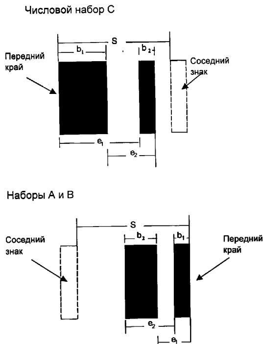
Рисунок 7 — Размеры декодирования знаков символов
