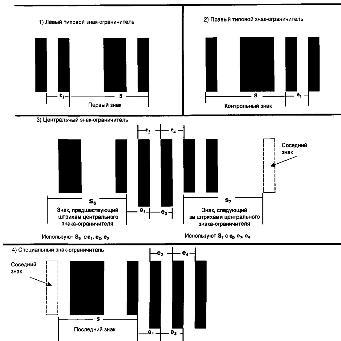
Рисунок 8 — Размеры вспомогательных знаков
