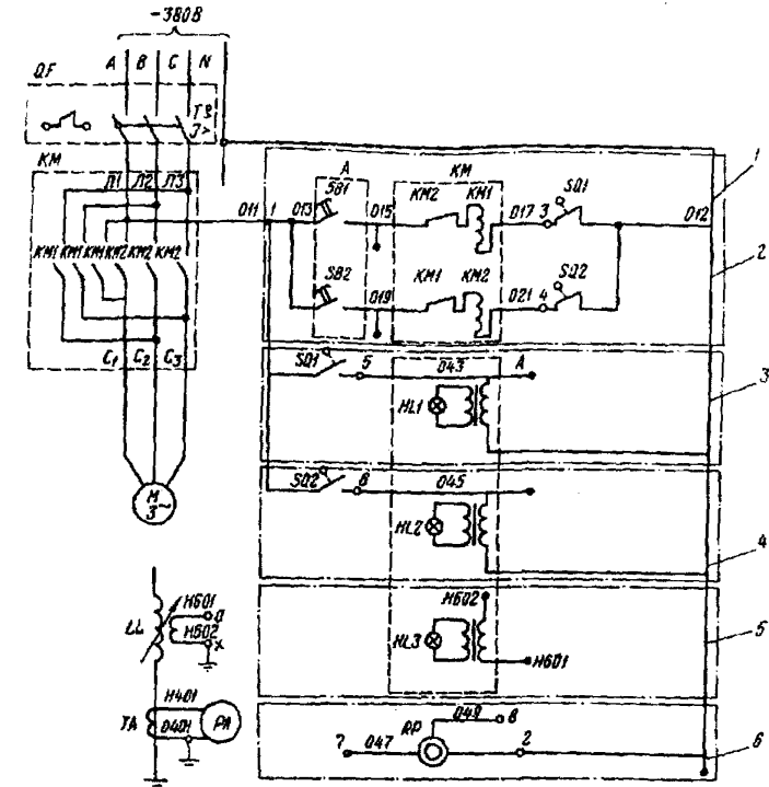
Рис.3. Электрическая схема управления электроприводом реакторов серии РЭДПМ:
