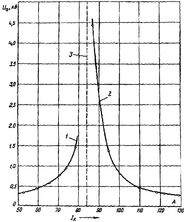
Рис. II. Кривая зависимости напряжения смещения нейтрали от настройки дугорасядающего реактора:
