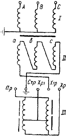
Рис.4. Электрическая схема дугогасящего устройства ТДЭТ-30/10:
