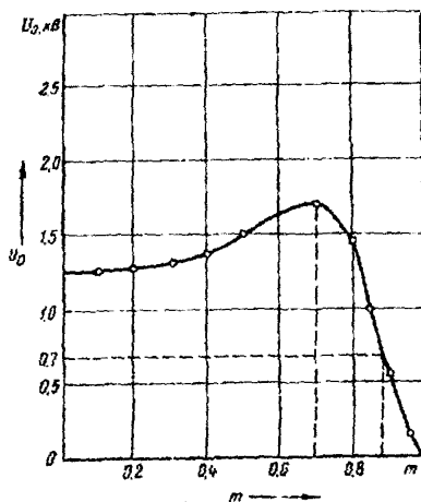
Рис.9. Кривая зависимости напряжения смещения нейтрали от степени однофазной несимметрии m
