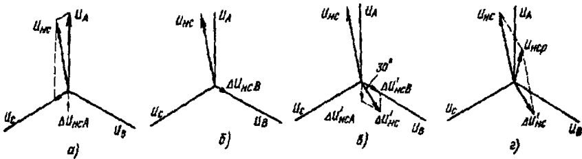
Рис.7. Изменение напряжения несимметрии сети при переносе конденсаторов высокочастотной связи с фазы А на фазу В U - изменение напряжения несимметрии при отключении конденсаторов на фазе А; б - изменение напряжения несимметрии при подключении конденсаторов на фазу В; в - суммарное изменение напряжения несимметрии; г - результирующее напряжение несимметрии
