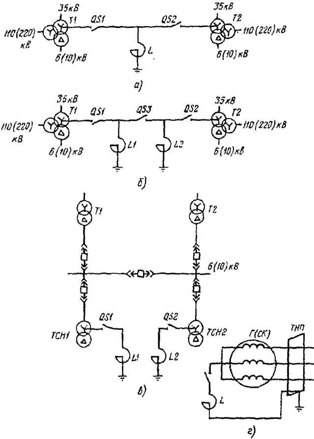
Рис.1. Схемы включения дугогасящих реакторов:
