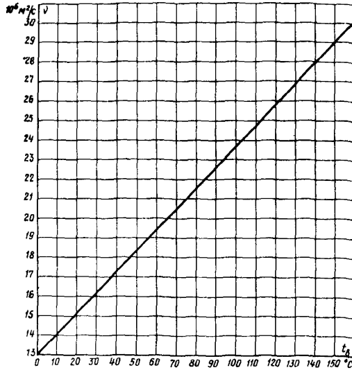
Рис. I7. Зависимость кинематической вязкости воздуха от температуры
