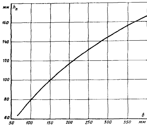
Рис.14. Зависимость высоты слоя аэропульты от ширины аэрожелоба
