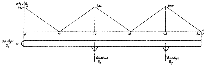
Рис.18. Эпюра распределения воздуха по длине аэрожелоба
