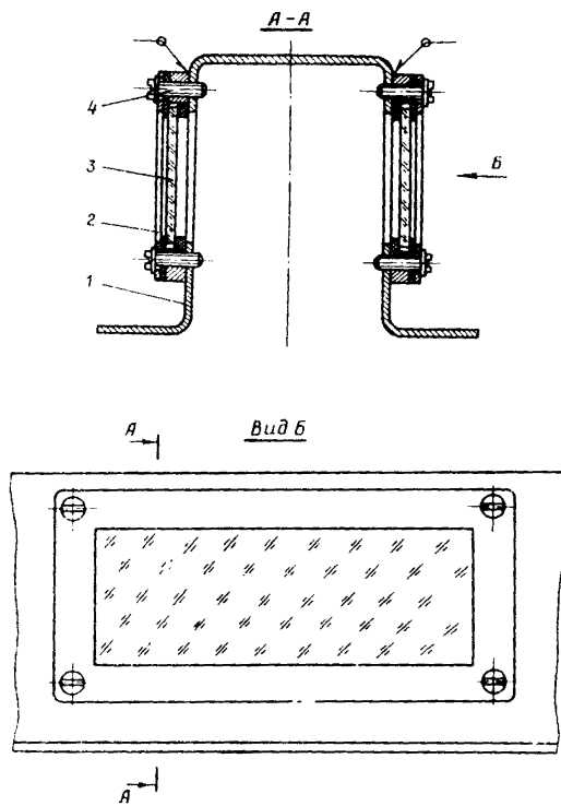
Рис.4. Смотровое окно: 1 - боковая стенка верхней камеры аэроже- лоба; 2 - прижимная рамка; 3 - стекло; 4 - винт
