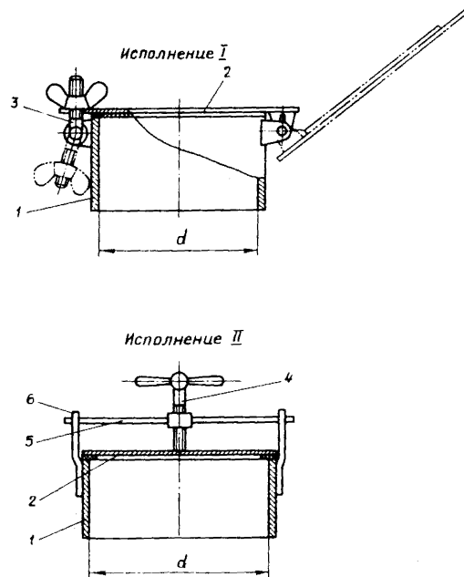
Рис.5. Продувочный лючок: I - корпус; 2 - крышка; 3 - откидной болт; 4 - винт; 5 - траверса; 6 - ушко
