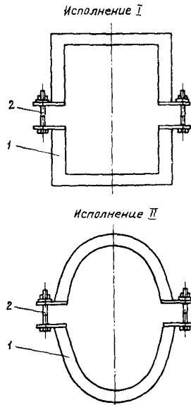
Рис.2. Зажим: I - скоба; 2 - болт
