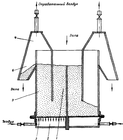
Рис. 13. Пневмослоевой переключатель:
