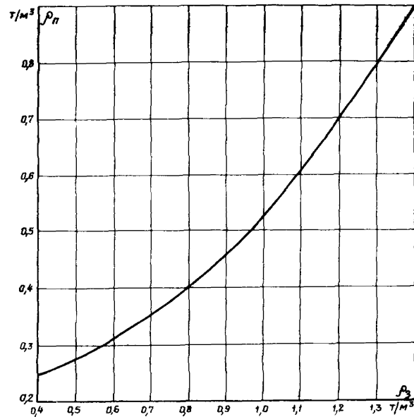
Рис.15. Зависимость плотности аэропульты от насыпной плотности золы
