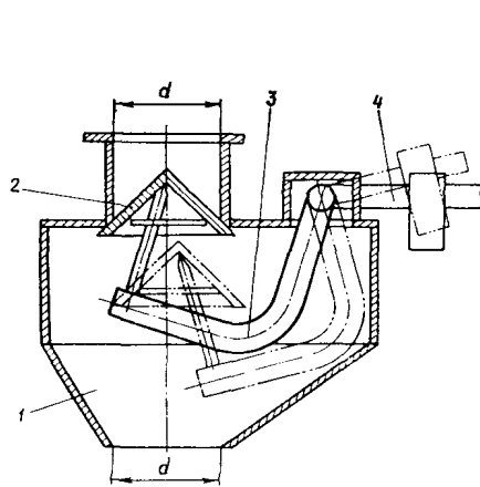
Рис.10. Мигалка:
