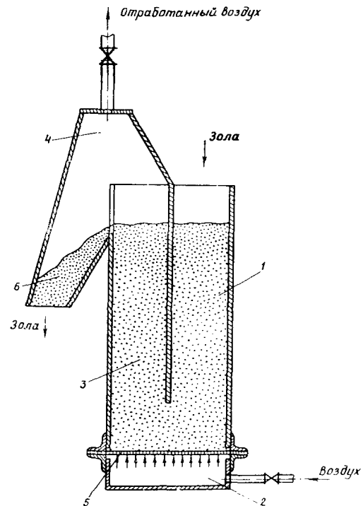
Рис.11. Пневмослойевой затвор:
