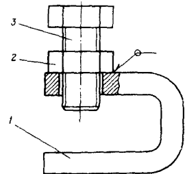
Рис.3. Струбцина: I - скоба; 2 - гайка; 3 - болт
