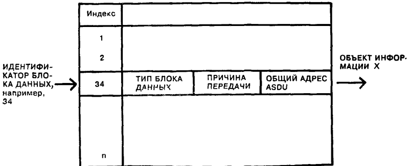
Рисунок 9 — Пример компактной идентификации ОБЪЕКТОВ ИНФОРМАЦИИ
