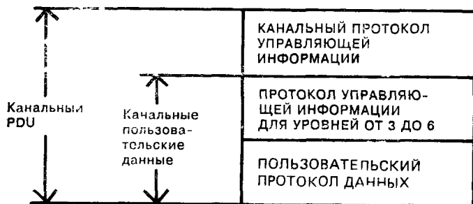
Рисунок 2 — Структура кадра для модели 1
