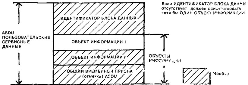
Рисунок 6 — Основная структура БЛОКА ПОЛЬЗОВАТЕЛЬСКИХ СЕРВИСНЫХ ДАННЫХ
