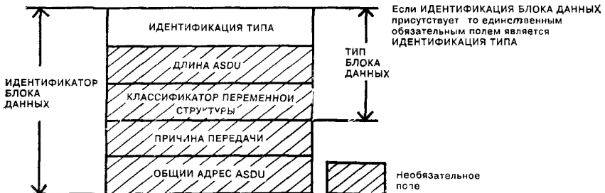
Рисунок 7 — Основная структура ИДЕНТИФИКАТОРА БЛОКА ДАННЫХ
