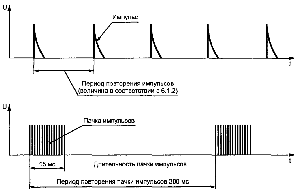
Рисунок 2 — Пачки НИП
