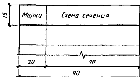
Ведомость перемычек
