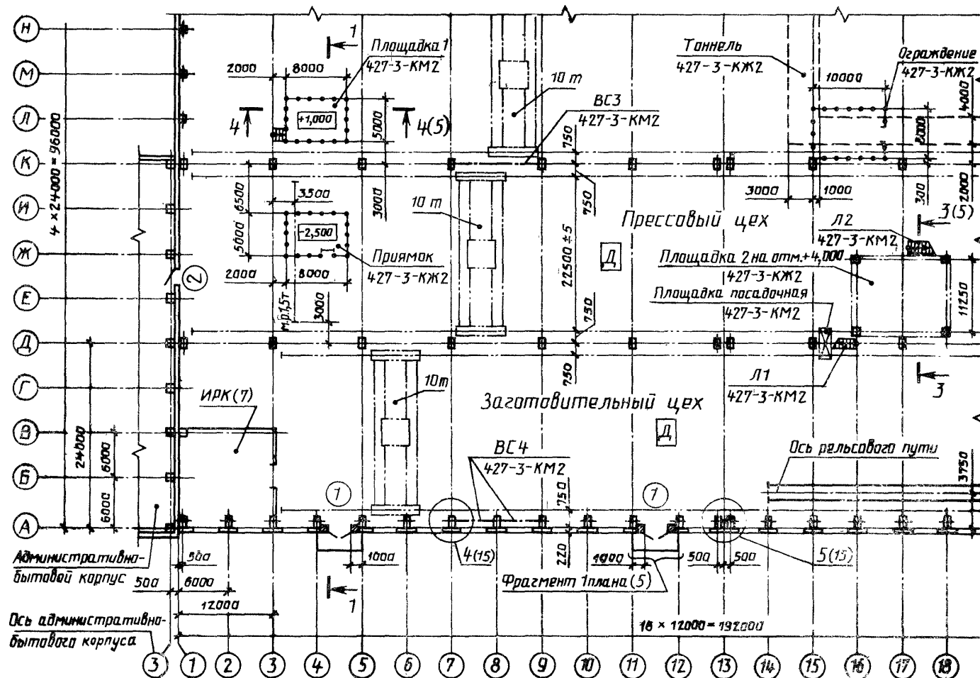
Пример выполнения плана одноэтажного производственного здания
