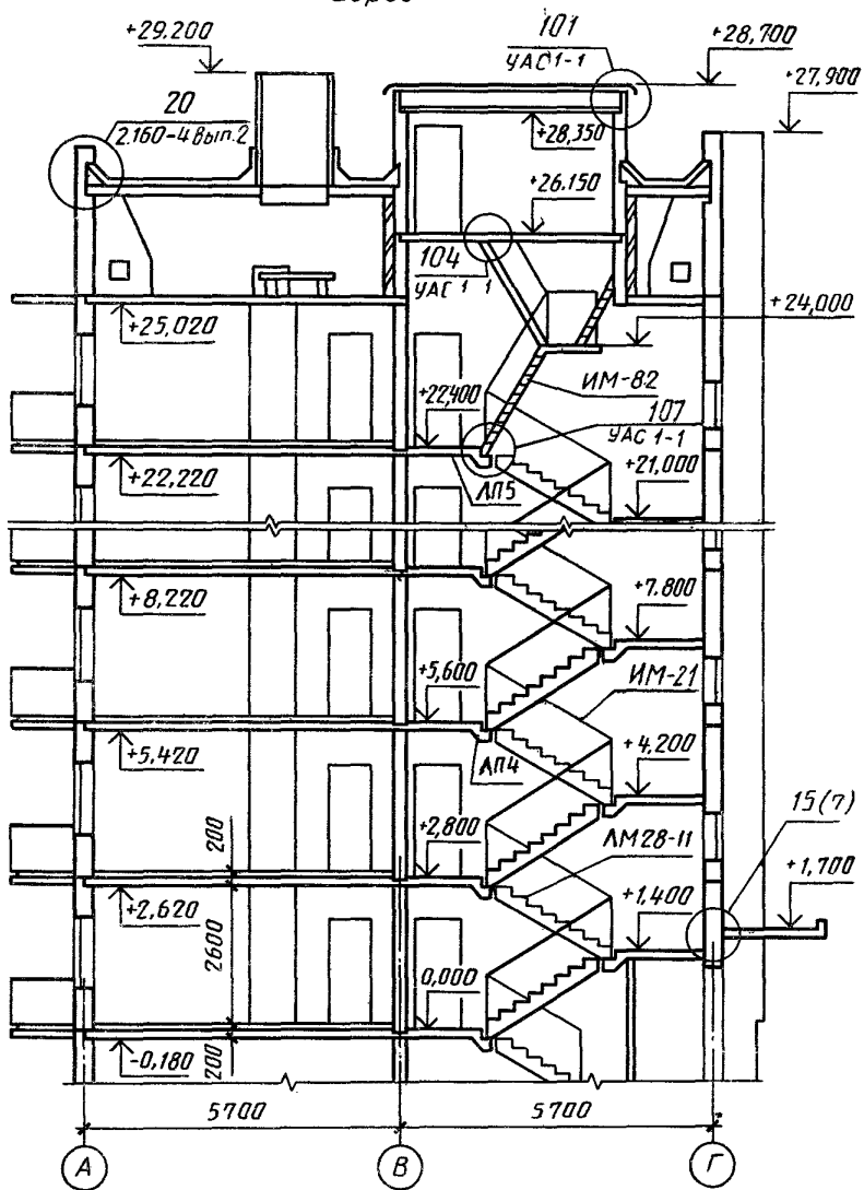
Разрез 1-1
