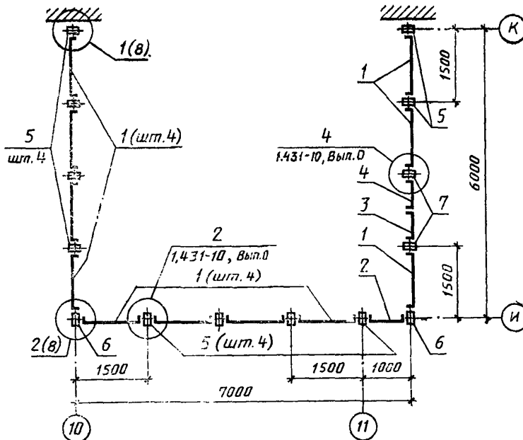
Пример выполнения схемы расположения элементов сборных перегородок
