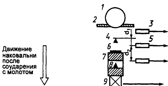
1 — молот; 2 — улавливающее устройство, 3 — фотодатчик запуска; 4 — нож в состоянии покоя; 5 — фотодатчик системы измерения скорости; 6 — прокладка; 7 — наковальня; 8 — светоотсекающий нож; 9 — калибруемый акселерометр
