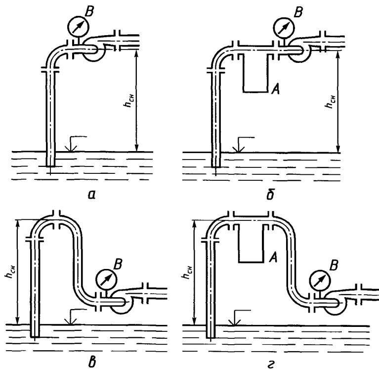
h_{сн} — номинальная высота самовсасывания; B — вакуумметр; A — емкость, имитирующая длинный горизонтальный участок всасывающего трубопровода
