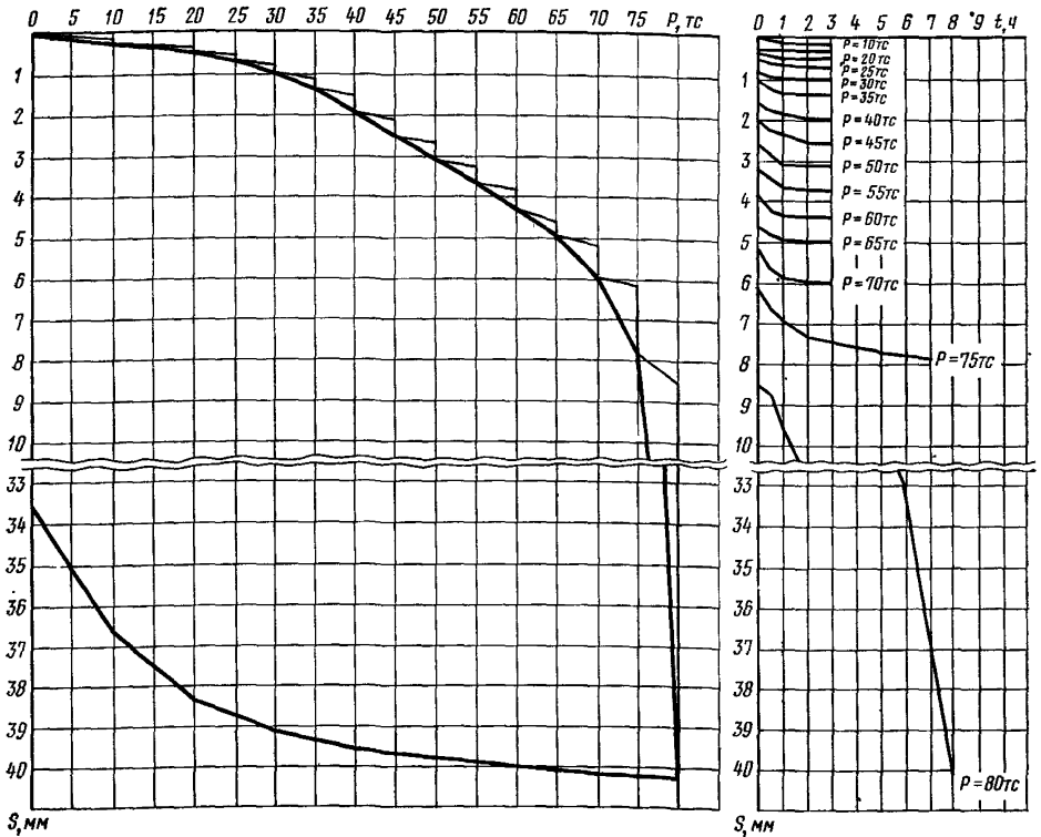
График изменения осадки сваи S во времени t (по ступеням нагрузки)
