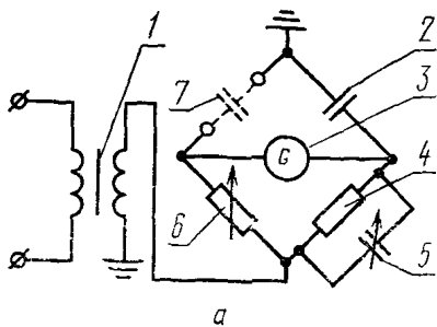
Схема с заземленной диагональю
