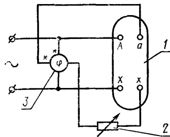
1—испытываемый трансформатор; 2—резистор регулируемый; 3—фазометр, А, X, а, x—зажимы испытываемого трансформатора.
