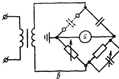
Схема с заземленной диагональю
