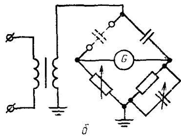
Схема с заземленной диагональю
