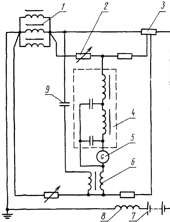
1—измеряемая обмотка; 2—регулируемый резистор; 3—резистор; 4—фильтр; 5—гальванометр; 6—трансформатор компенсирующий; 7—аккумуляторная батарея; 8—дрозель; 9—разделительный конденсатор
