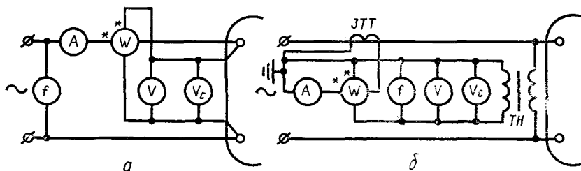
При включении приборов через измерительные трансформаторы тока и напряжения
