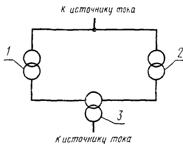
1—испытуемый трансформатор; 2—вспомогательный трансформатор; 3—трансформатор
