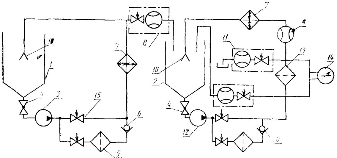
Схема испытательного стенда для определения характеристик фильтрования
