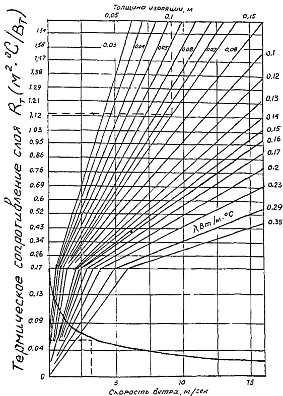
Рис. 9. Номограмма для определения термического сопротивления теплоотдаче опалубки в зависимости от расчетной скорости ветра и термических сопротивлений слоев опалубки соответствующих толщин и коэффициентов теплопроводности
