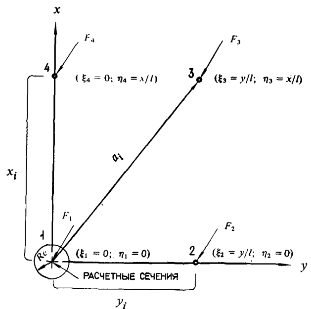
Черт. 2. Расчетная схема параметров загрузки опор воздушного судна
