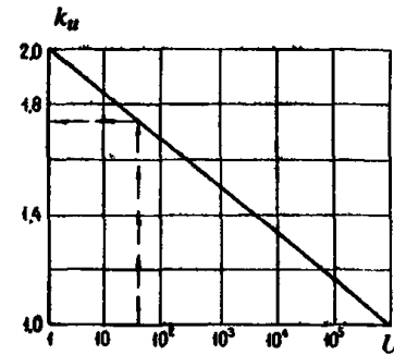
Черт. 3. График для определения коэффициента k_u
