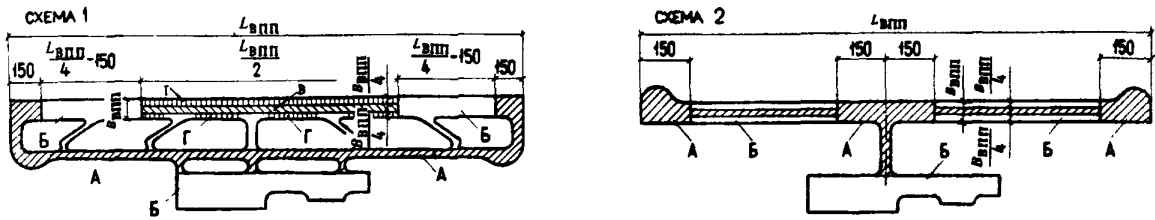
Черт. 1. Схемы деления покрытий аэродрома на группы участков
