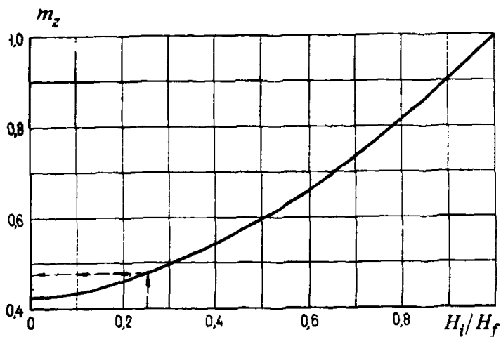
Черт. 2. График для определения коэффициента m_z
