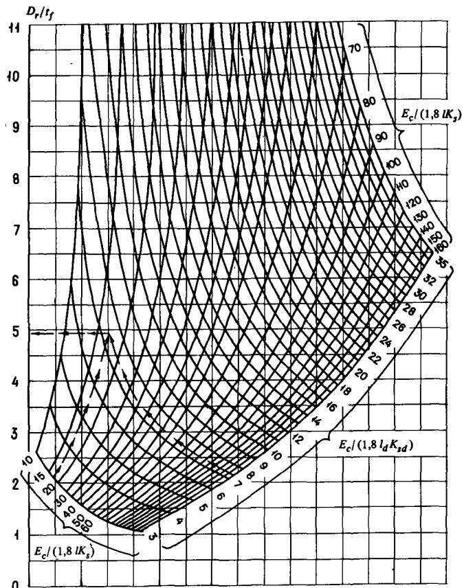
Черт. 2. Номограмма для определения отношения \frac{D_r}{t_f}
