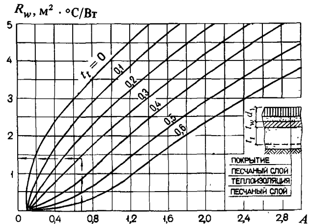
Черт. 2. Номограмма для определения термического сопротивления теплоизоляции
