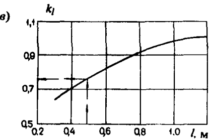
Черт. 1. Значения переходных коэффициентов k а — для положительных изгибающих моментов; б — для отрицательных изгибающих моментов; в — график для определения поправочного коэффициента k_l к переходному коэффициенту k
