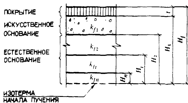
Черт. 1. Расчетная схема слоистого основания
