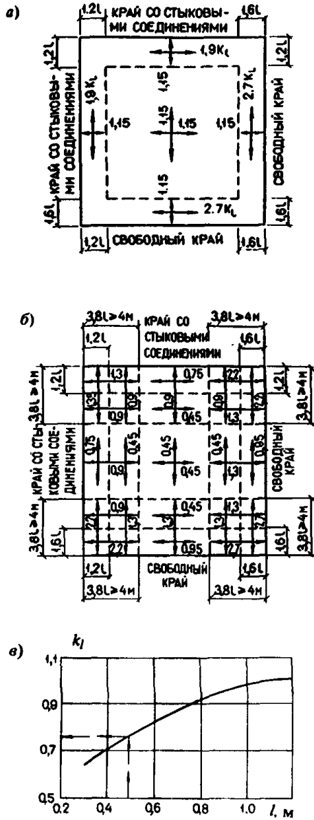
Черт. 1. Значения переходных коэффициентов k а — для положительных изгибающих моментов; б — для отрицательных изгибающих моментов; в — график для определения поправочного коэффициента k_l к переходному коэффициенту k
