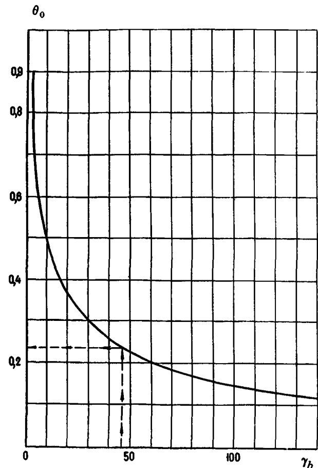
Черт. 1. График для определения \theta_0
