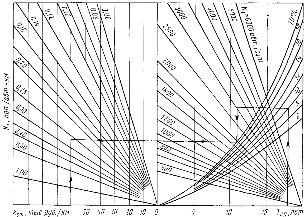
Рис. 4. Номограмма для определения удельных капиталовложений K_1 : при ежегодном приросте интенсивности движения по геометрической прогрессии с убывающими темпами роста
