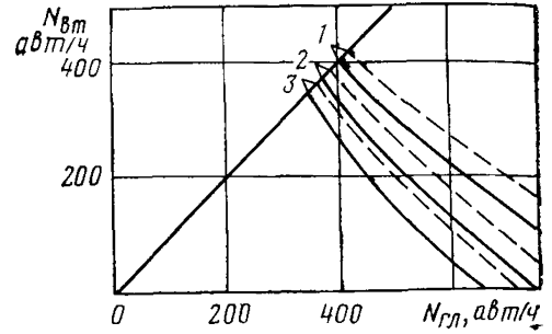
Рис. 3.7. Номограмма для определения пропускной способности нерегулируемых пересечений в одном уровне: 1 — теоретическая; 2 — максимальная практическая; 3 — практическая. Сплошные линии — необорудованные пересечения, штриховая — канализованные
