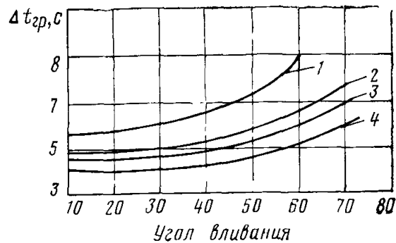
Рис. 4.2. Влияние угла вливания на критический промежуток времени:
