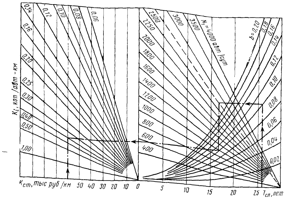
Рис. 2. Номограмма для определения удельных капиталовложений при ежегодном линейном приросте интенсивности движения ( K_{ст} — приведенная за T_{сл(t)} стоимость строительства одной полосы проезжей части, тыс. руб./км)
