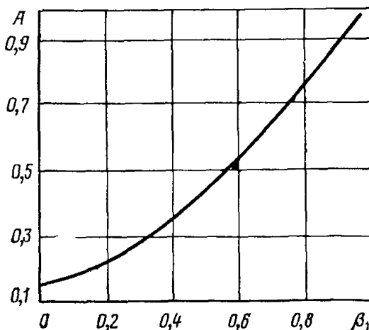
Рис. 3.5. Зависимость между коэффициентами А и B_1
