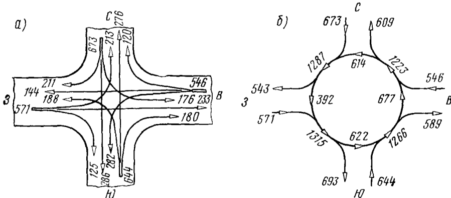
Рис. 3.9. Картограмма интенсивности движения:
