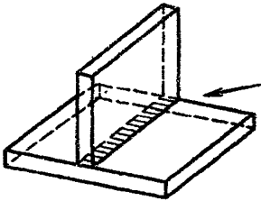
Рис.9. Нижнее положение
