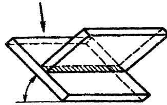
Рис.8. Положение "в лодочку"
