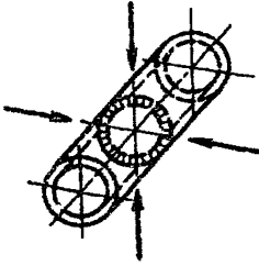
Рис.7. Переменное положение при горизонтальном расположении оси труб, свариваемых без поворота
