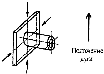
Рис.14. Переменное положение при горизонтальном расположении оси трубы, привариваемой без поворота
