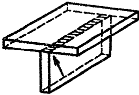
Рис.11. Потолочное положение
