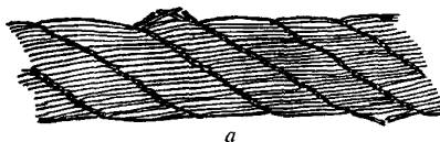
Рис. 1. Обрывы и смещения проволок каната крестовой свивки
