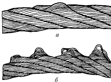
Рис. 11. Выдавливание проволок прядей: a — в одной пряди; б — в нескольких прядях
