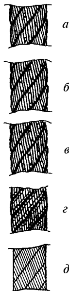
Рис. 4. Износ наружных проволок каната крестовой свивки: а — небольшие лыски на проволоках; б — увеличенная длина лысок на отдельных проволоках; в — удлинение лысок в отдельных проволоках при заметном уменьшении диаметра проволок; г — лыски на всех проволоках, уменьшение диаметра каната; д — интенсивный износ всех наружных проволок каната (уменьшение диаметра проволок на 40 %)
