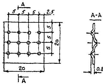
Рис.5. Схема соединения пластмассовых труб для электропроводок с помощью царапающей вставки:
