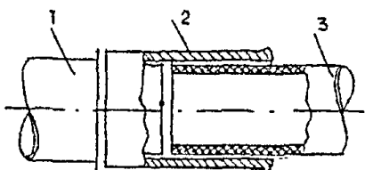
Рис.8. Схема соединения стальной с пластмассовой трубой для электропроводок: 1—стальная труба; 2—стальная (чугунная) муфта; 3—пластмассовая труба
