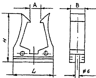
Рис. 10. Схема пластмассовых ящиков типа Л 75УЗ-Л178УЗ для крепления пластмассовых труб для электропроводок
