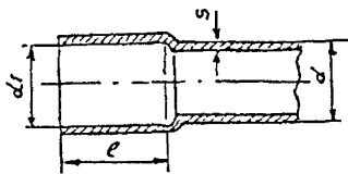
Рис.1 Схема раструба на пластмассовой трубе для электропроводок
