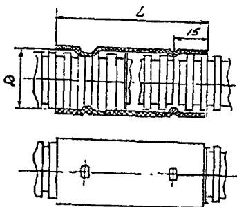
Рис. 17. Схема соединения пластмассовых гофрированных труб для электропроводок посредством муфты с выступами:
