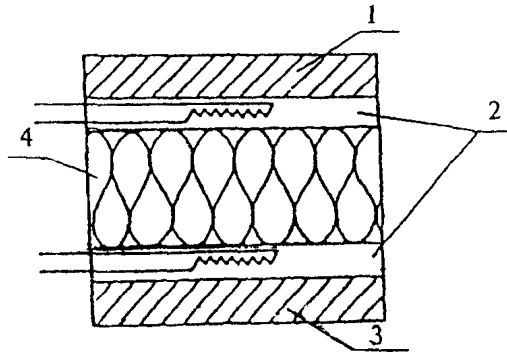
Рисунок А.2 — Схема прибора с двумя тепломерами
