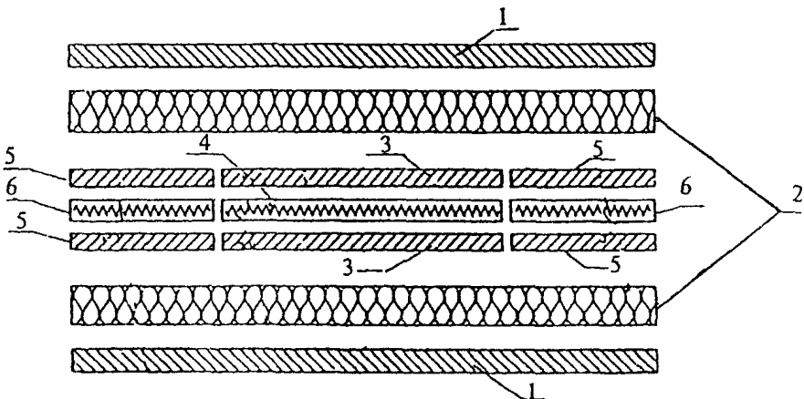
Рисунок А.2 — Схема прибора с двумя тепломерами
