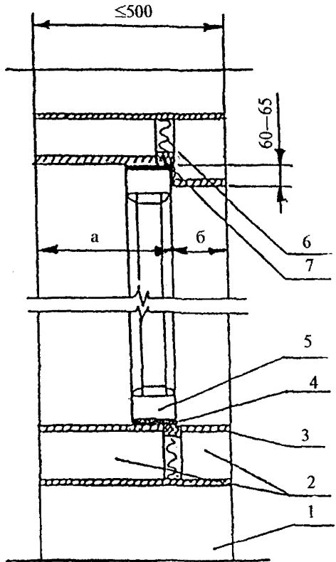
Вариант с многослойной перегородкой
