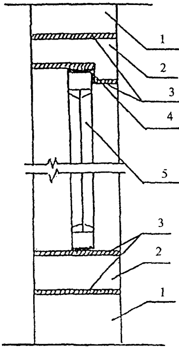
Вариант с однослойной перегородкой
