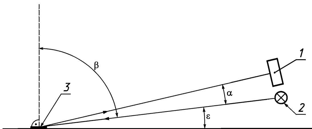
1 — фотоприемник; 2 — источник света; 3 — поверхность разметки; \beta = 87,7^\circ ; \alpha = 0,95^\circ ; \varepsilon = 1,34^\circ
