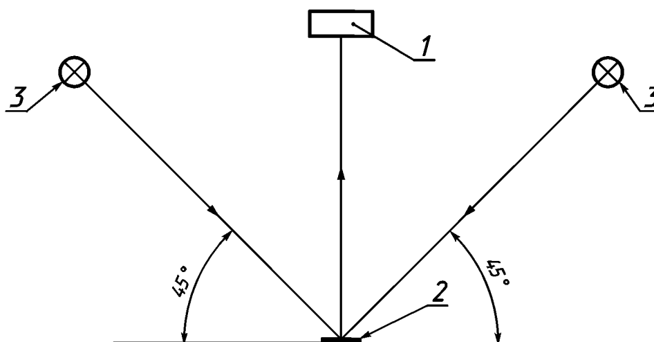
1 — спектрофотометр или колориметр; 2 — дорожная разметка; 3 — источник света
